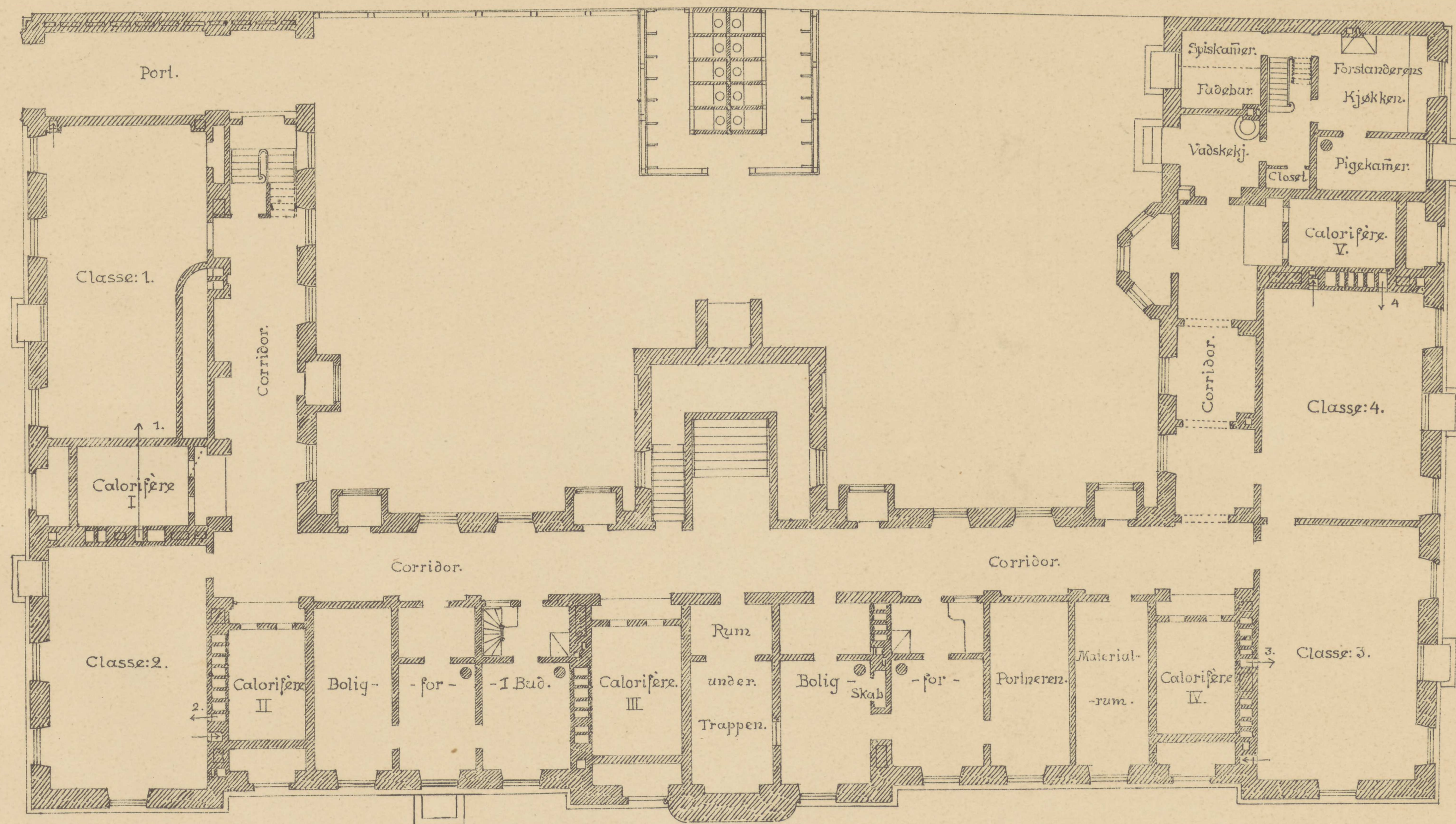
Plan af øversig Kjælder.
