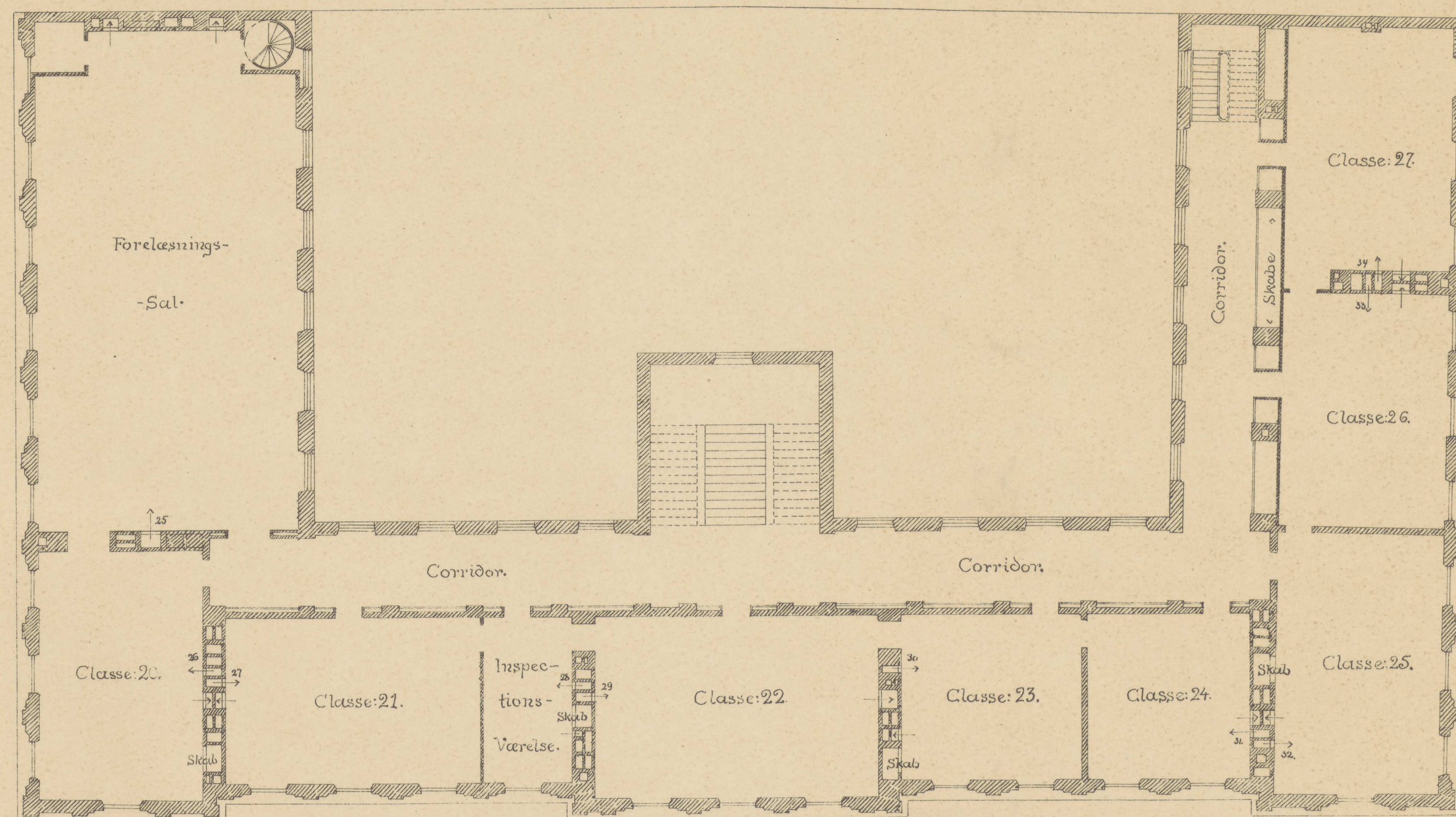
Plan af 2den Sal.
