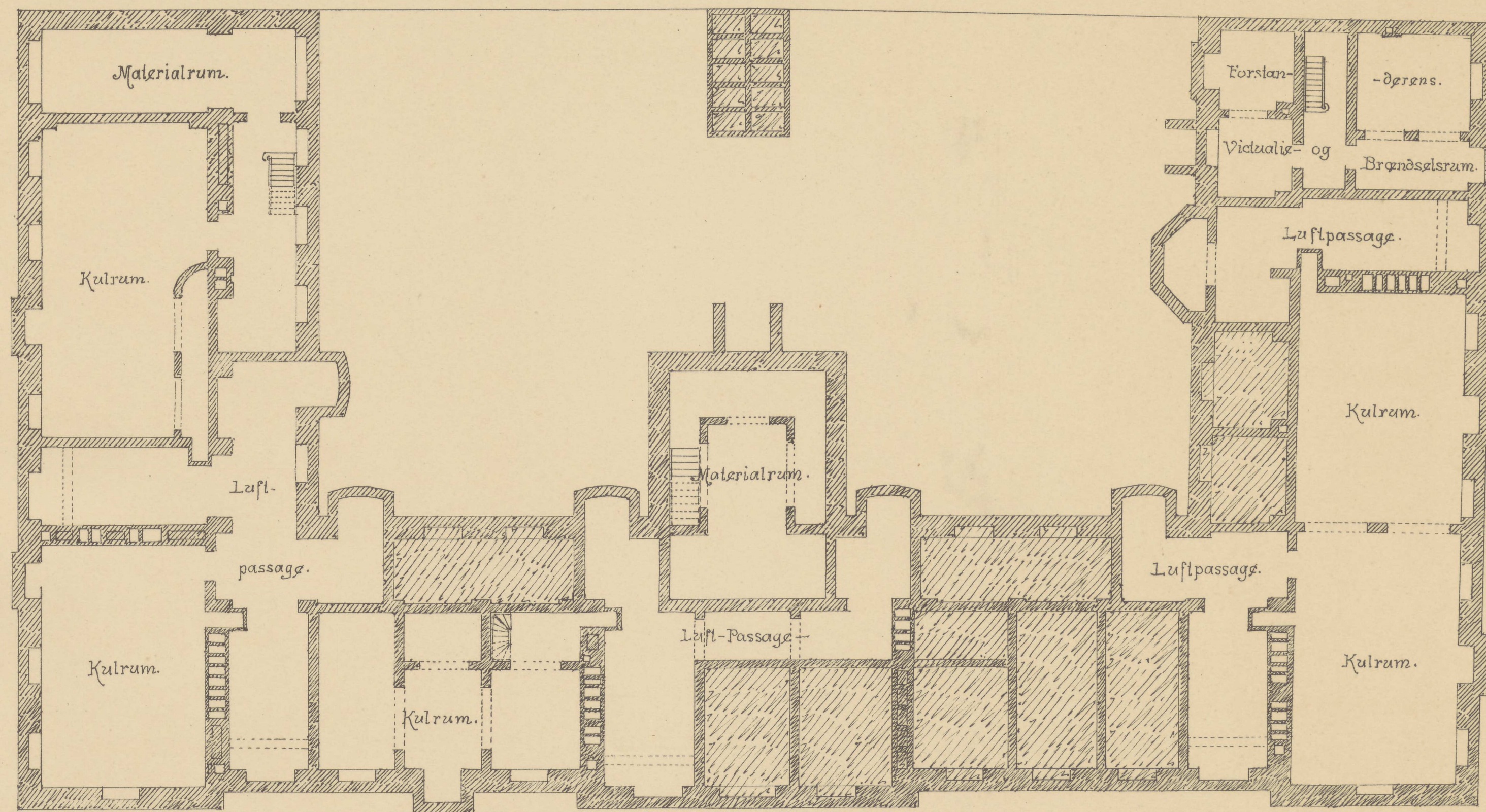
Plan af underste Kjælder.
