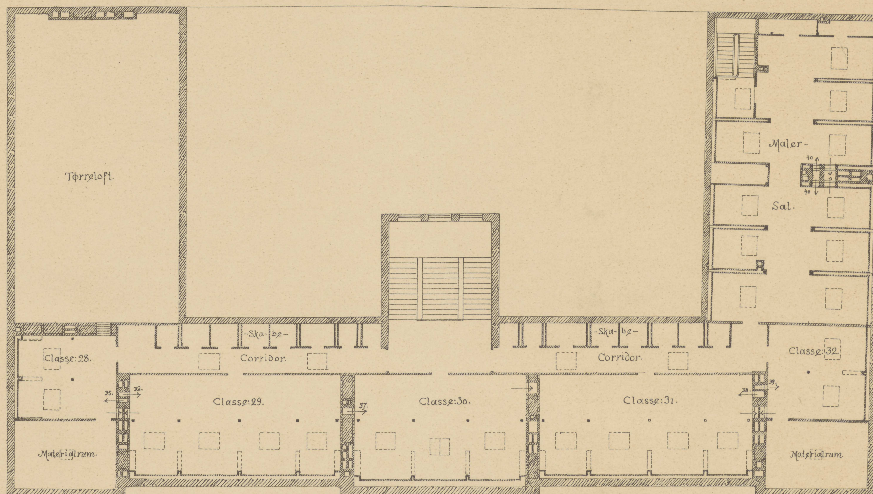
Plan af Tagelaget.
