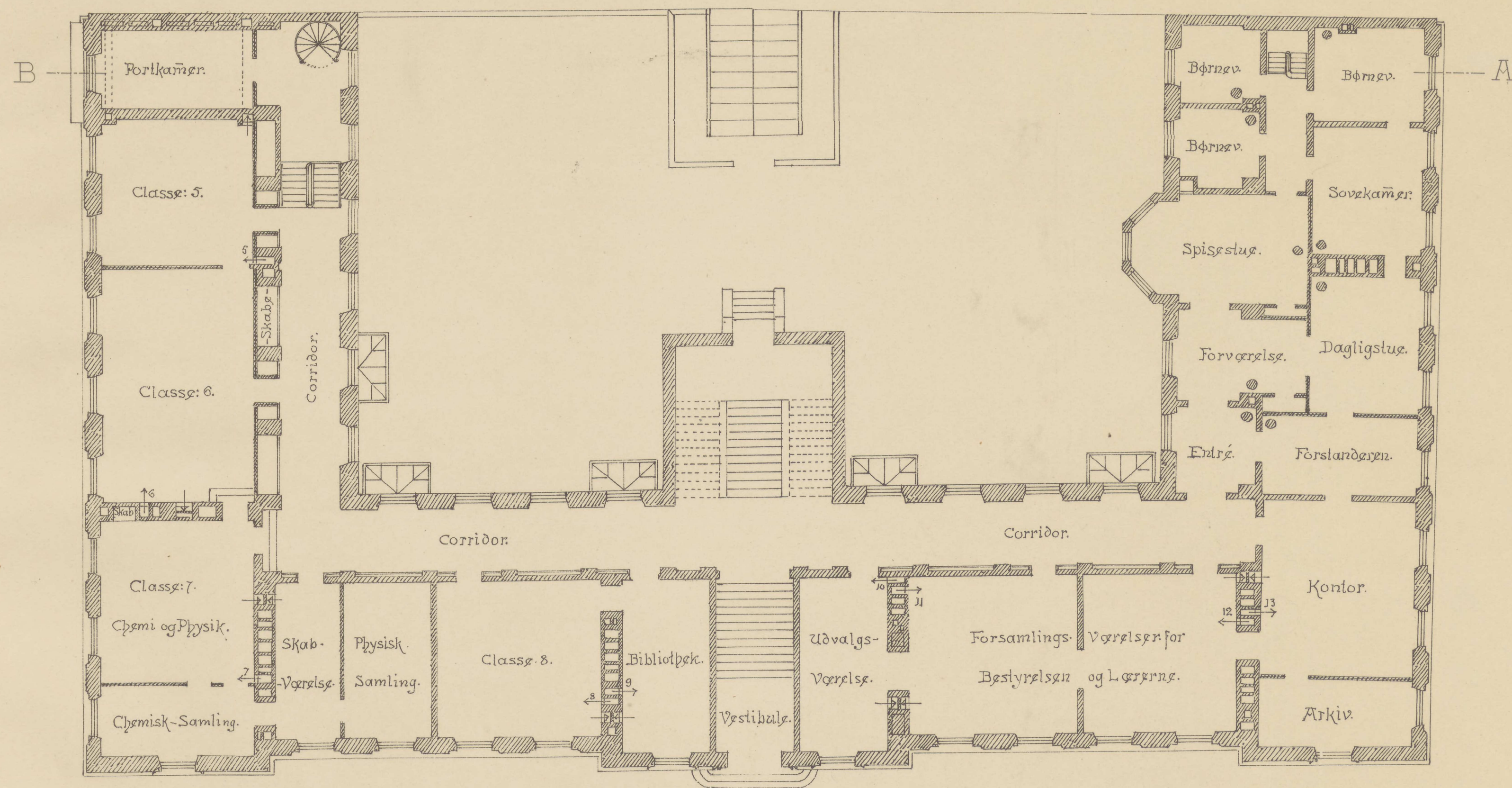
Plan af Stuen.
