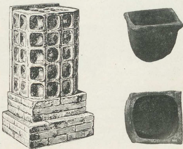
Fig. 81. Potteovn i Folkemuseet. (Efter Feilberg; Dansk Bondeliv).
