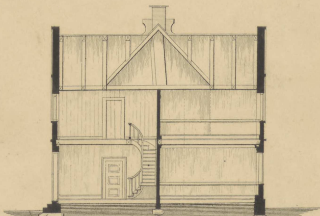
Profil efter AB.
