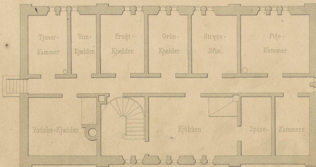
Plan af Kjælder-Etagen.
