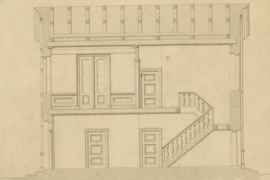
Profil efter Linien A.B.
