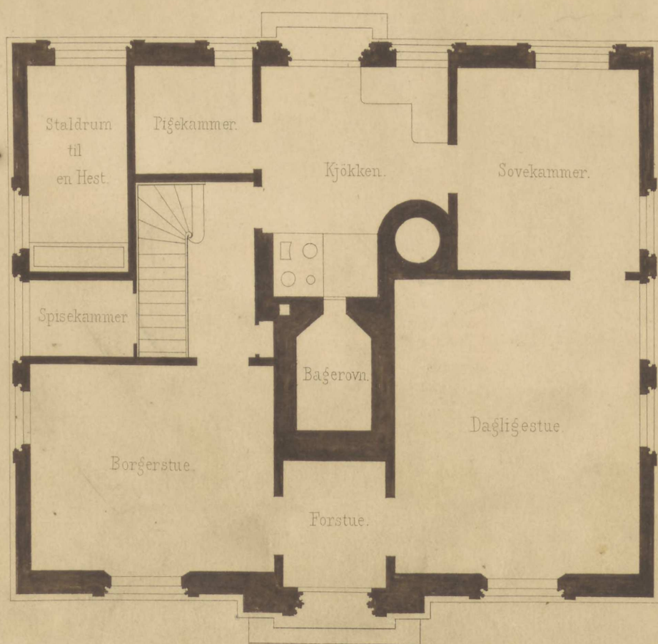
Plan.
