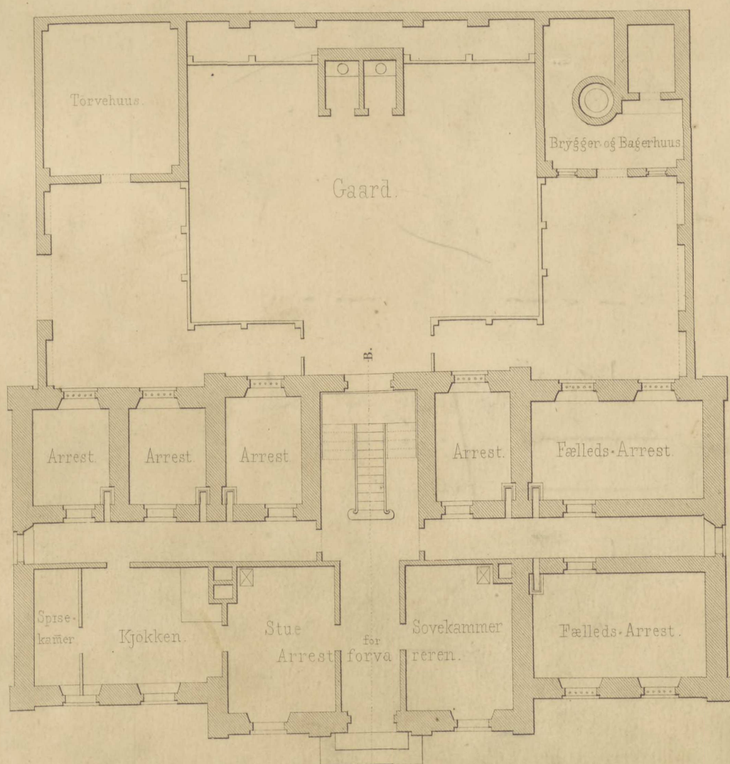
Plan af 1 ste Etage.
