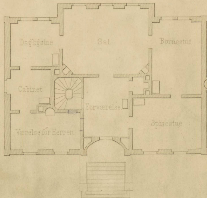
Stue Etage.
