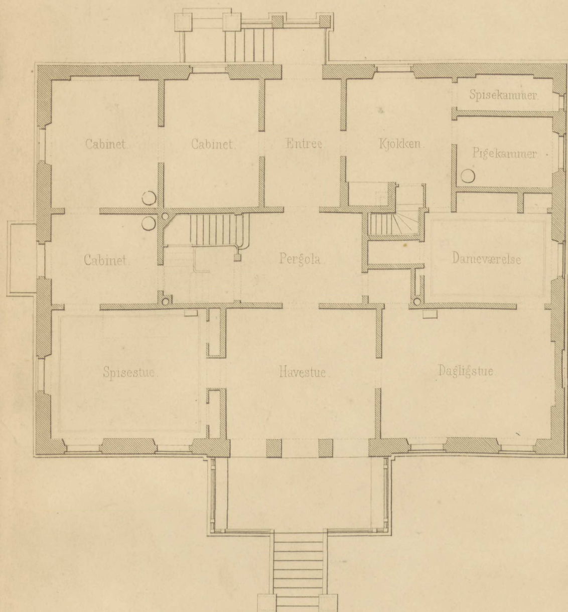
Plan af den øverste Etage.
