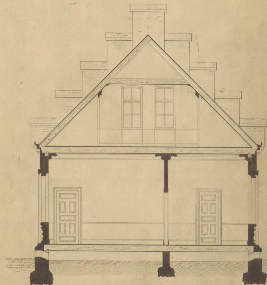
Tverprofil.
