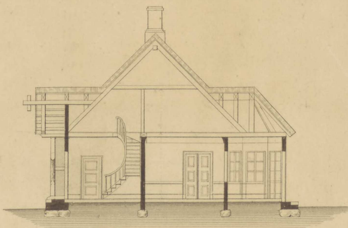
Profil efter AB.
