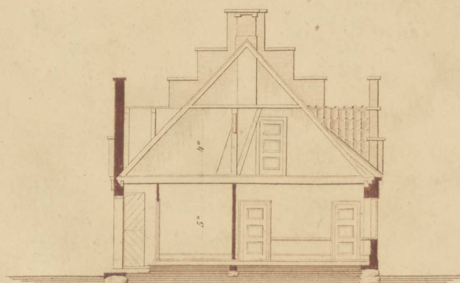
Profil efter AB.
