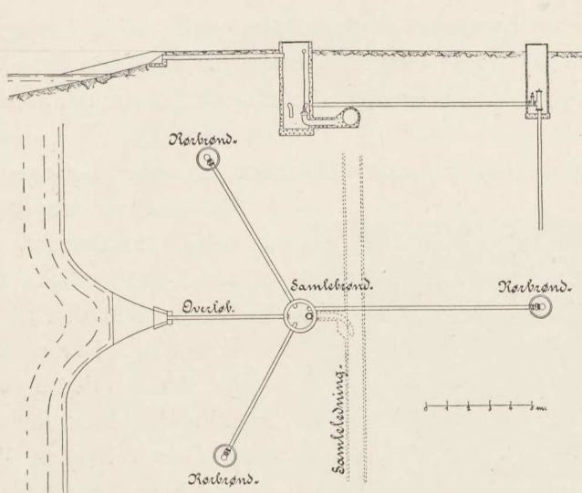
Samlebrønd med Boringer ved Søndersø.
