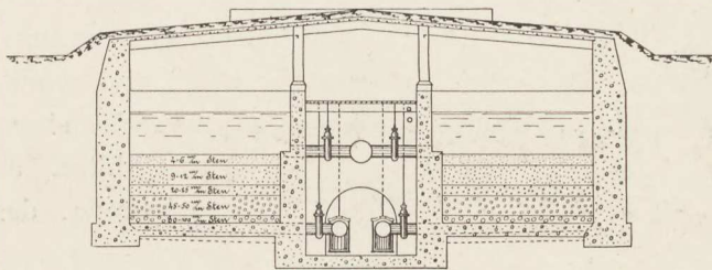
Tværsnit af Afgjæringsfiltret, Borups Allé.
