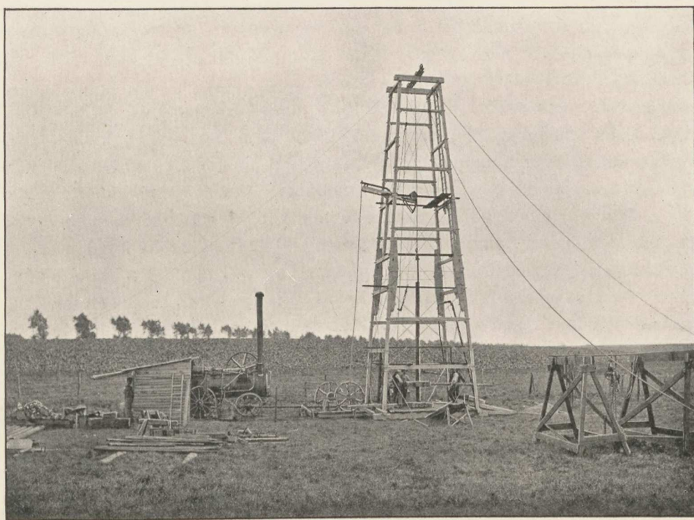
Vandværkets Boretaarn.
