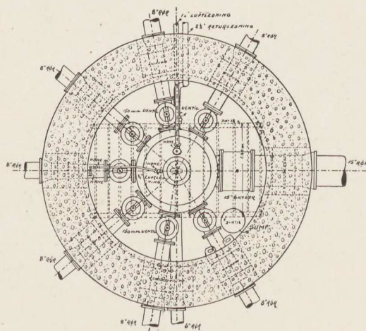
Solhøj Huse, Forbindelsen mellem en Gruppe Børinger og Samleledningen.
