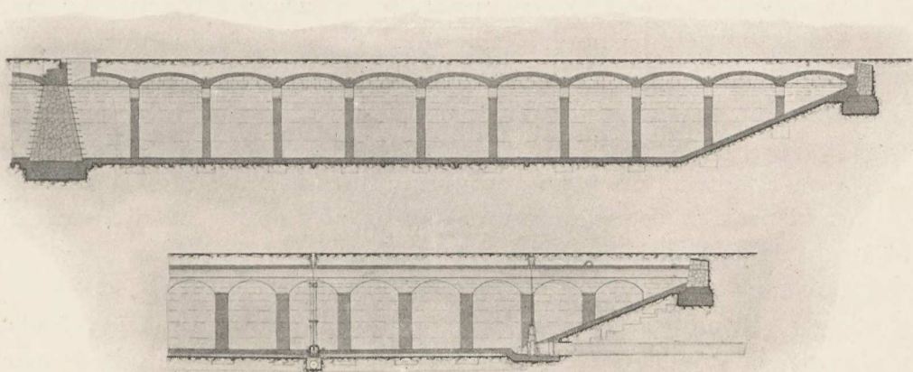
Søndermarksbassinet efter Overdækningen.
