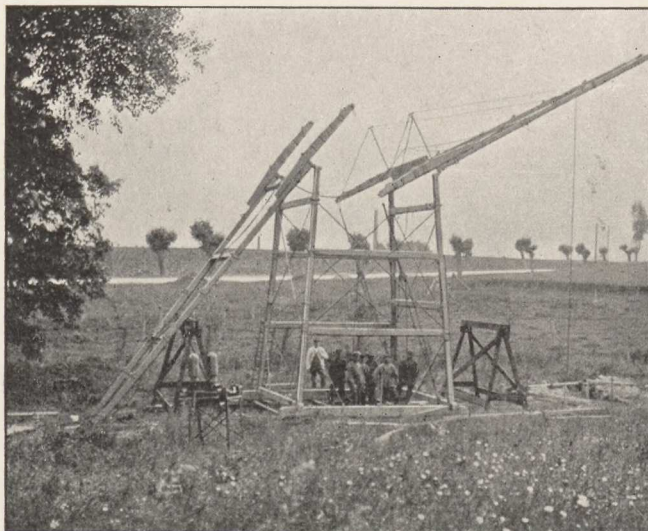
Boretarnet rejses.
