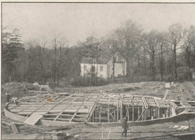
Vandreservoiret ved Thorsbro under Udførelsen.
