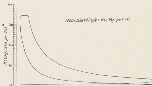
Indikatorgram fra Dieselmotorerne.
