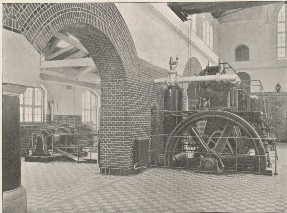
Maskinsalen ved Thorsbro, Dieselmotor med Højtrykscentrifugalpumpe.
