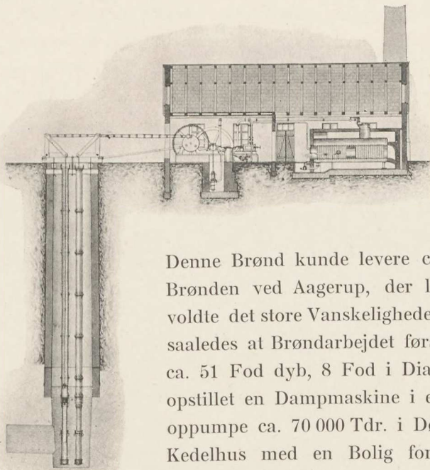
Brøndanlæg ved Kildeplads Nr. 10.
