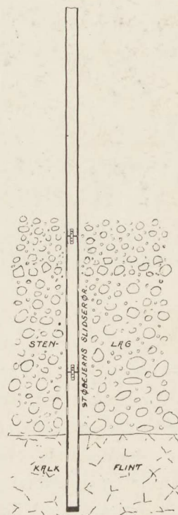
Type paa Boring ved Søndersø.
