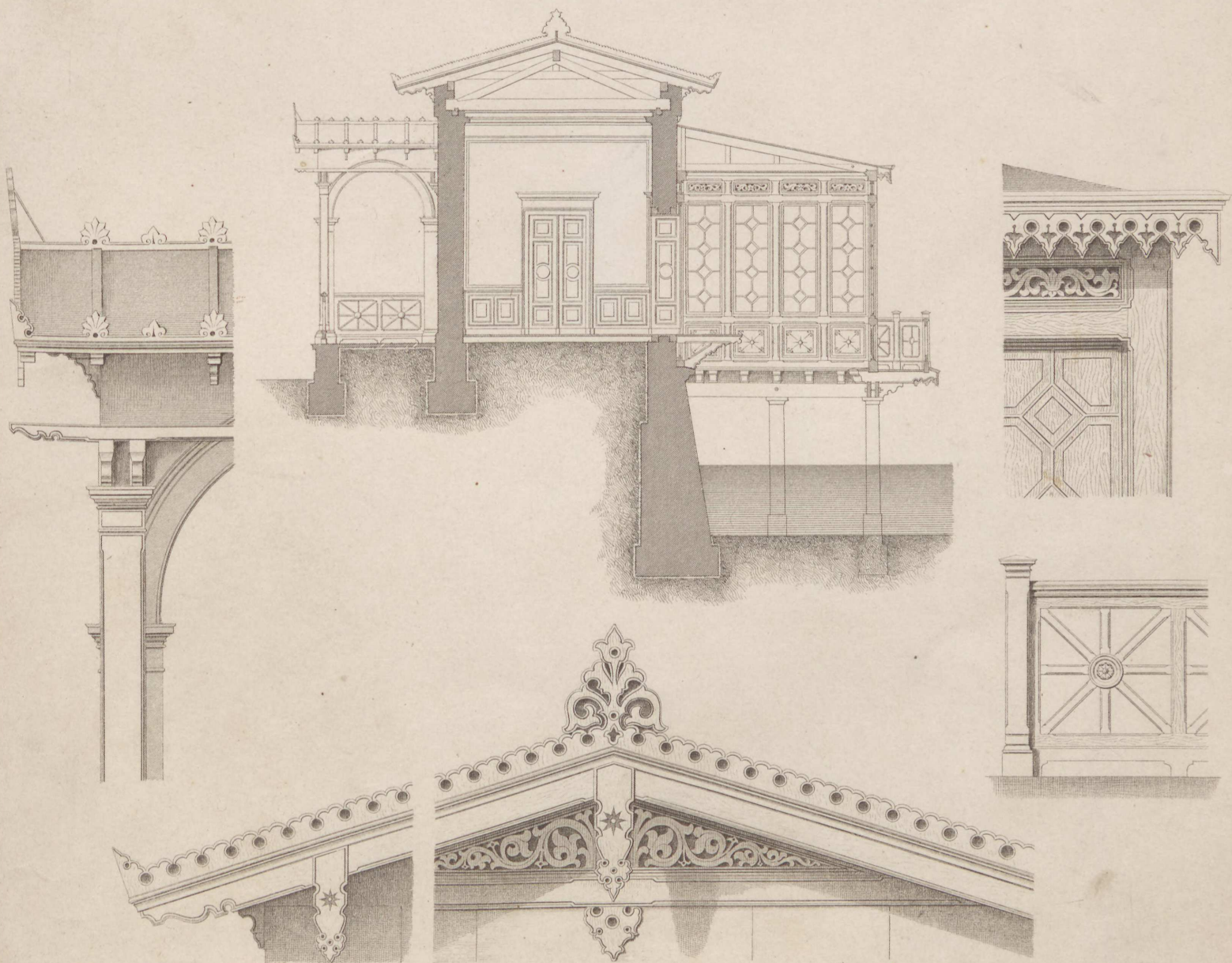
Badehäuschen im Park des Schloßes Albrechtsberg bei Dresden.
