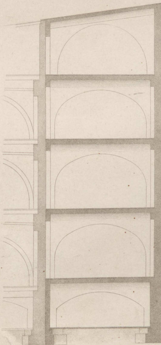
Querschnitt a-b.
