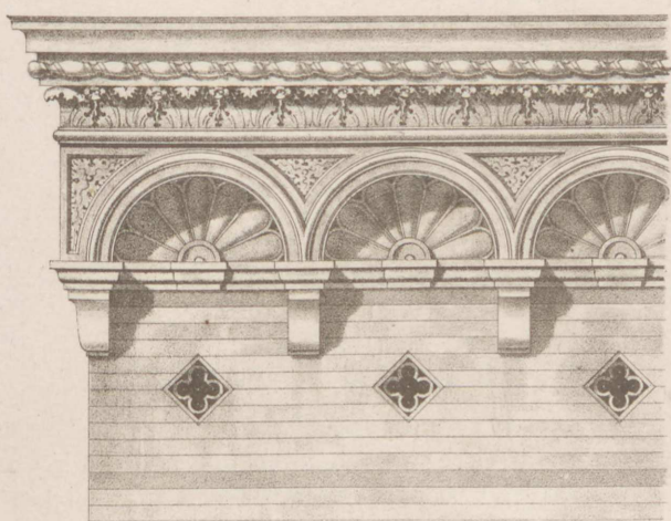
Hauptgesims des Wohngebäudes.
