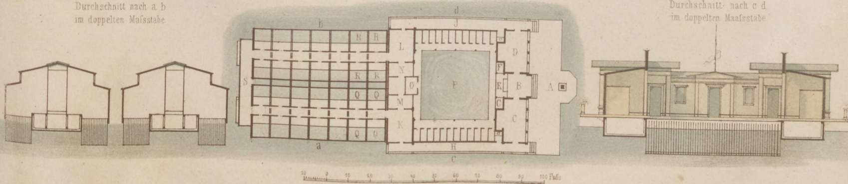
Strombad des Herrn Louis Sintenis in Magdeburg.
