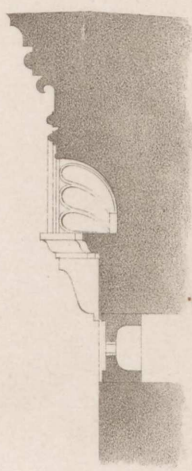
Profil.
