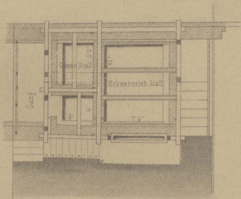
Grundriss.
