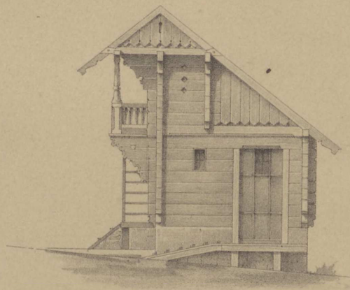
Giebel Ansicht.
