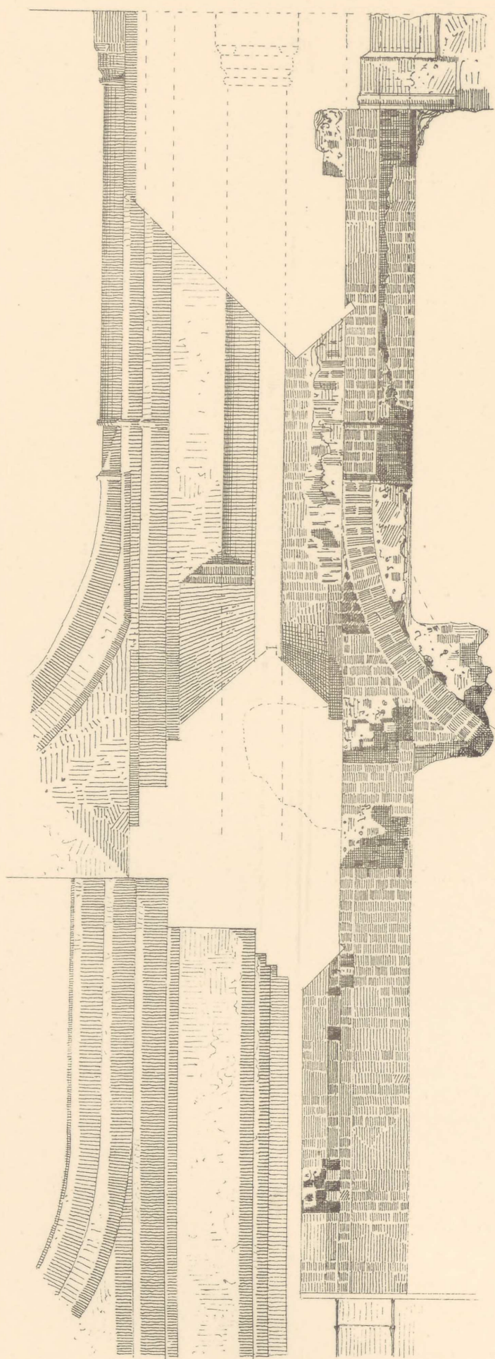
ENKELTHED AF SNIT C—D. SE BLAD XXIII.
