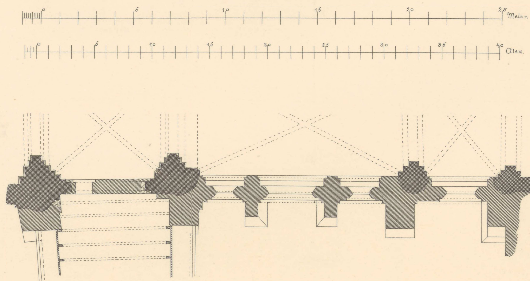
SNIT G—H.
