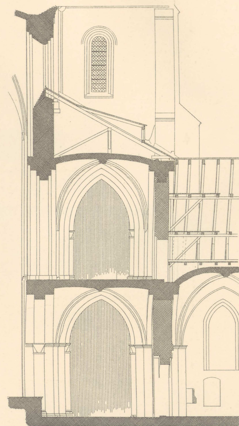
SNIT G—H.
