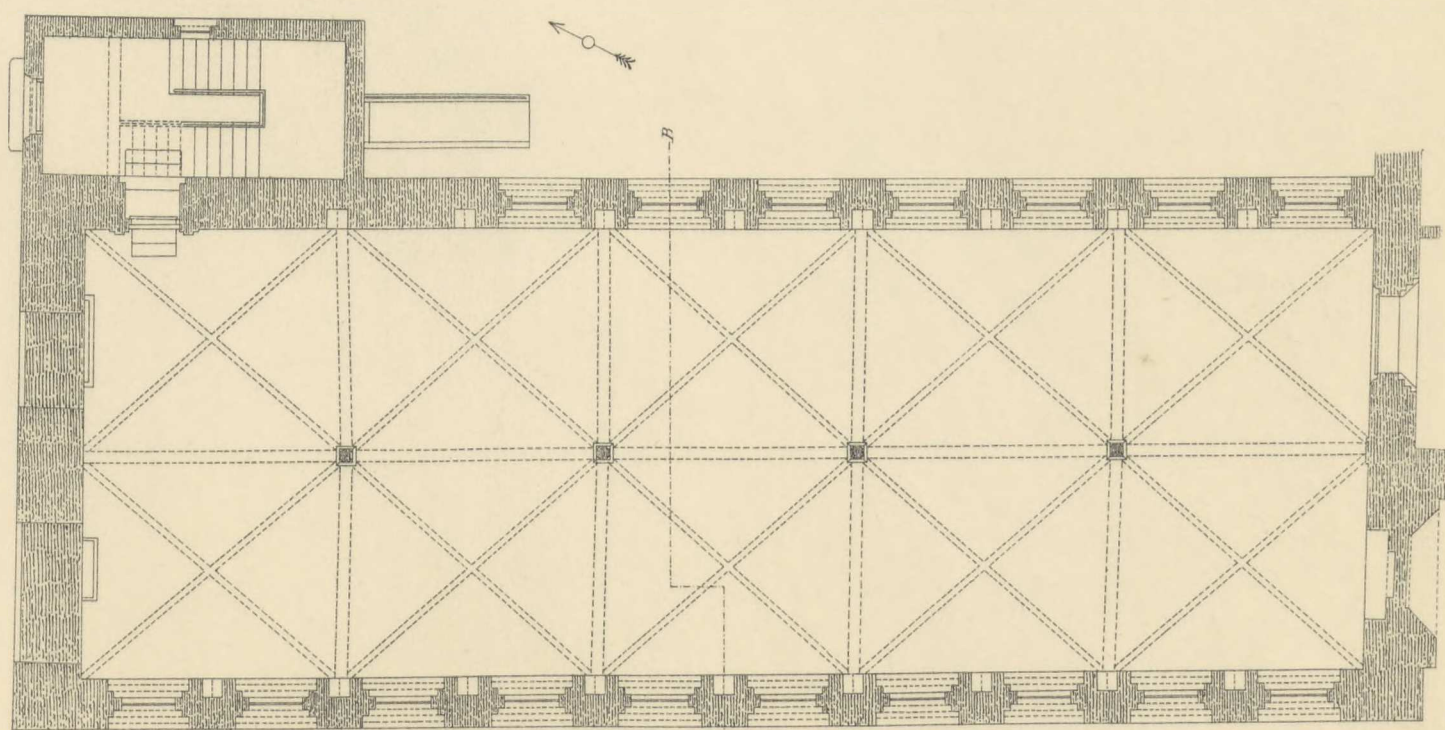
STUEPLAN
