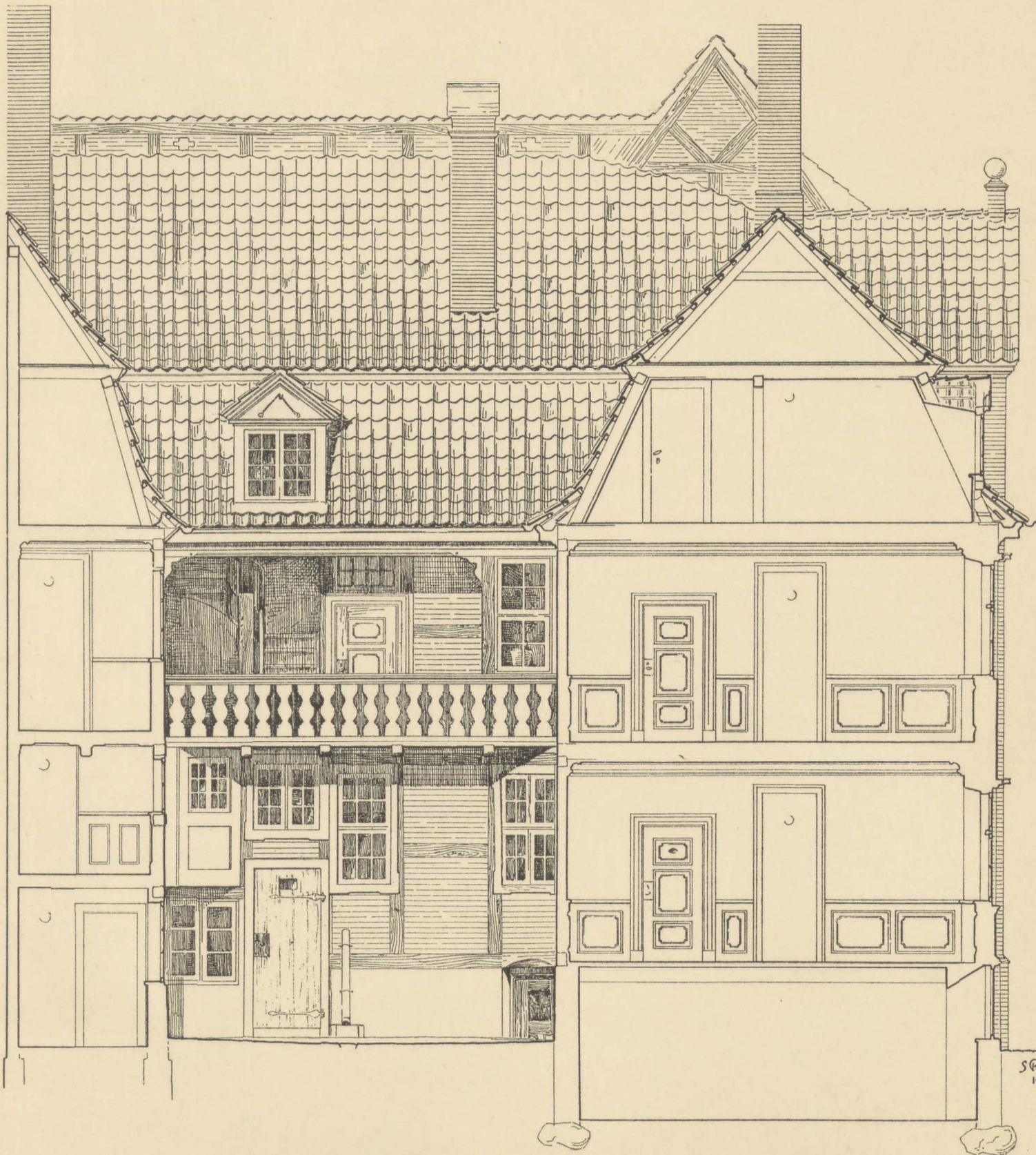
SNIT GENNEM GAARDEN.
