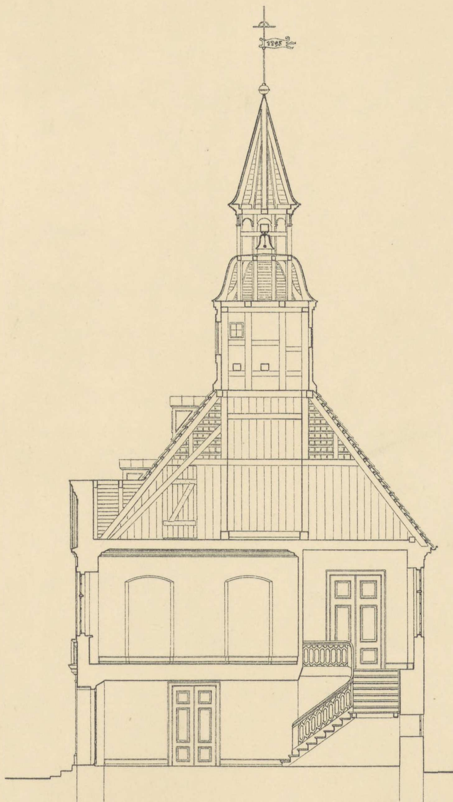
TVÆRSNIT
