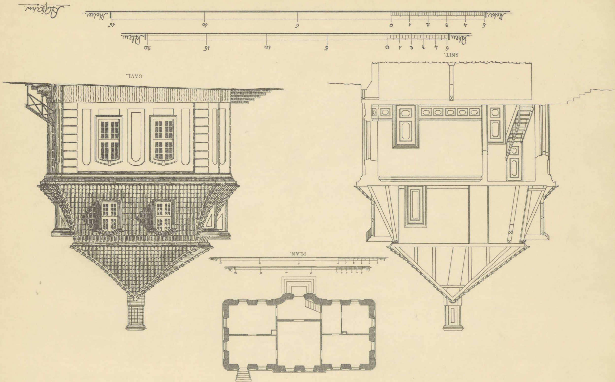
INGEMANNNS HUS I SORØ.
