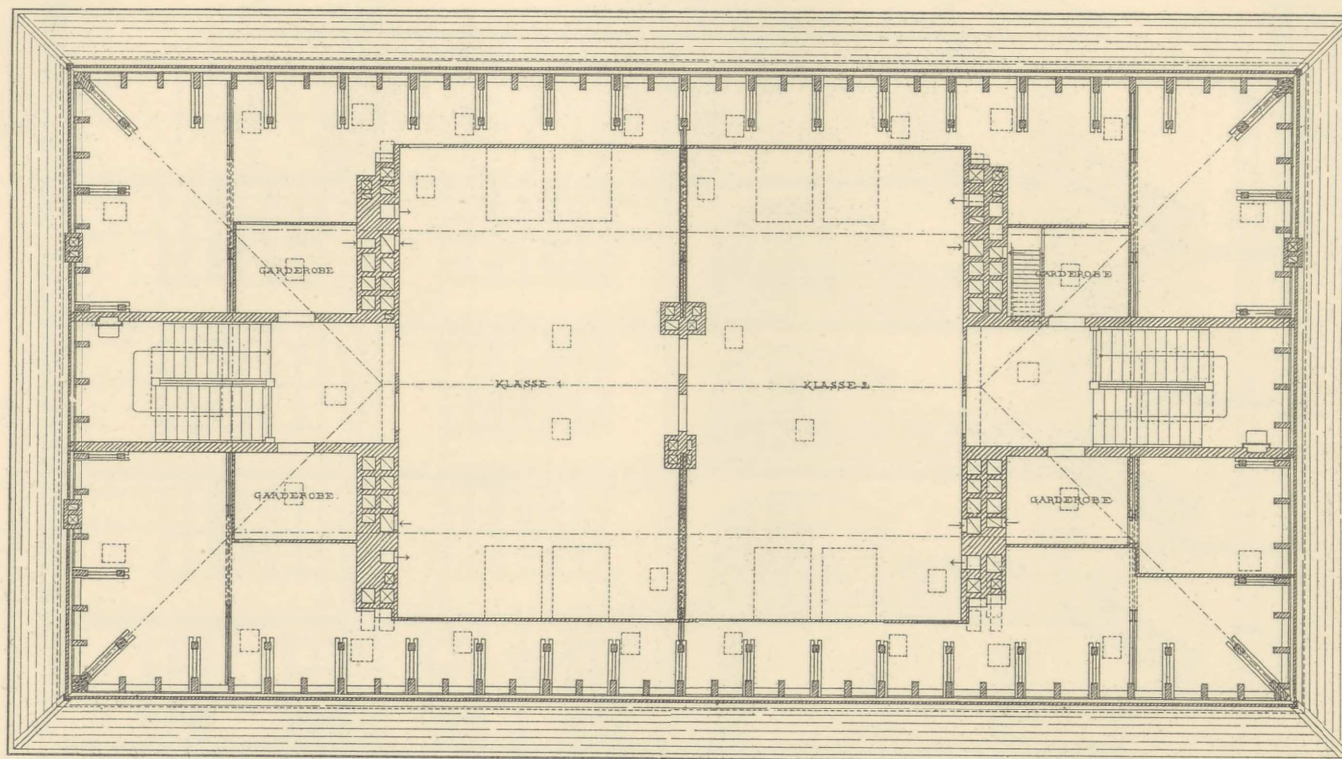
• TAGPLAN •
