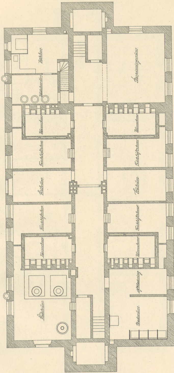
• KÆLDERPLAN •
