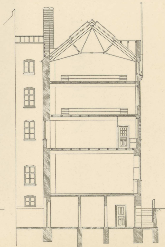
TVÆRSNIT
