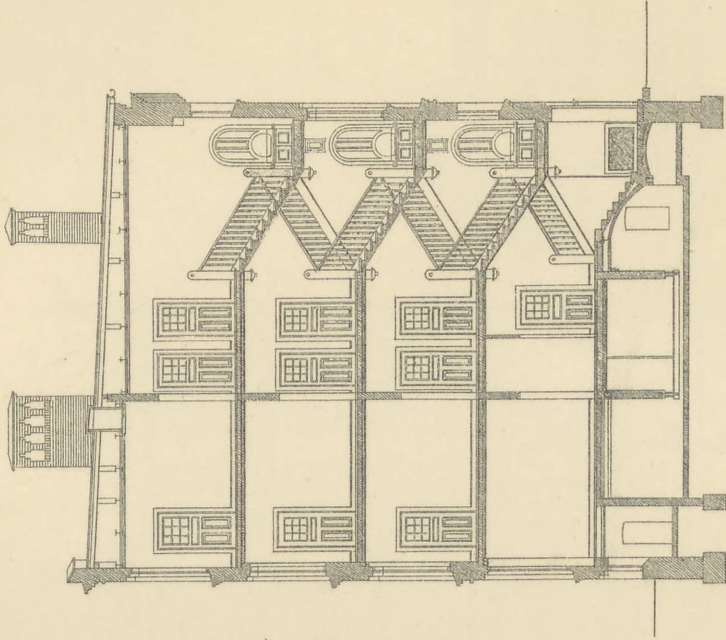
Stueplan.
