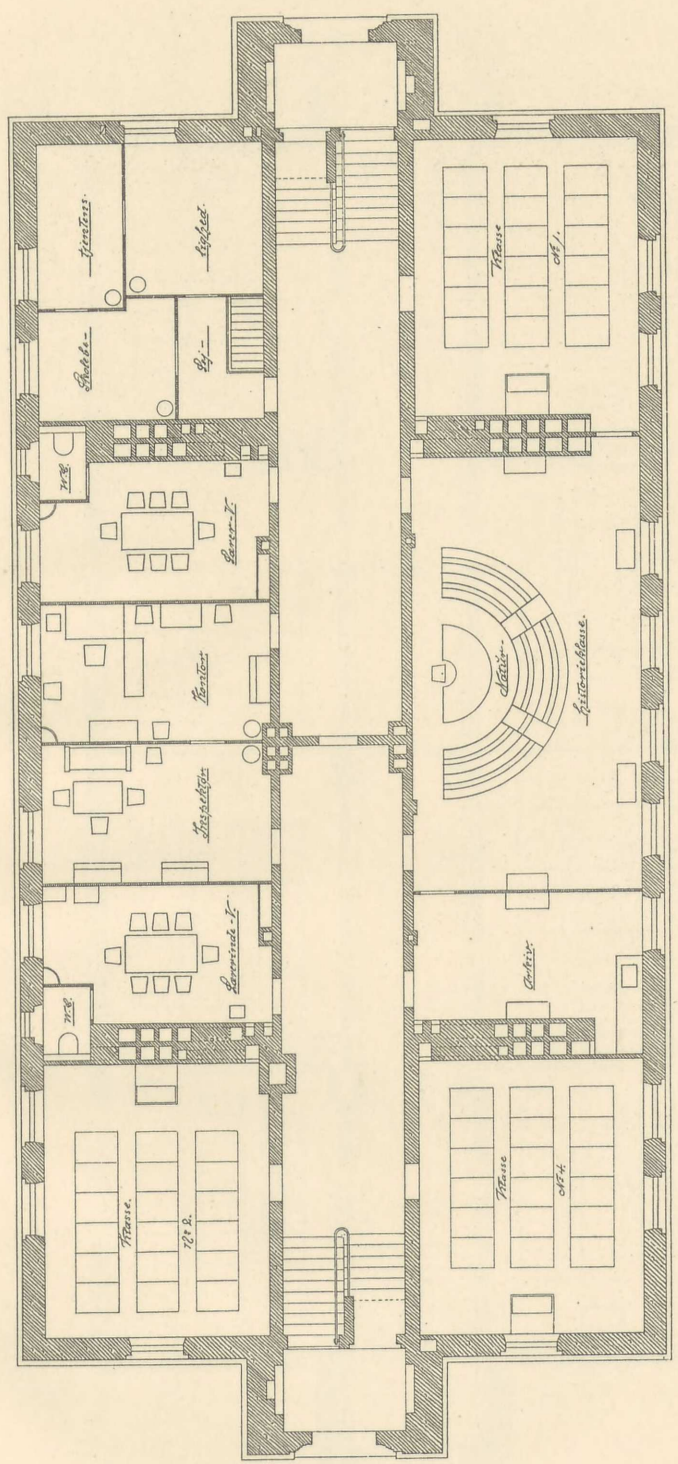
• STUEPLAN •
