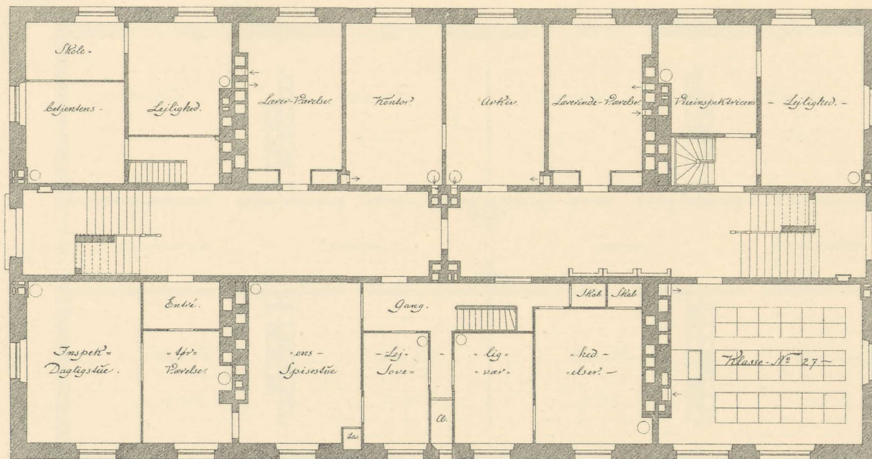
Plan af Skolen.
