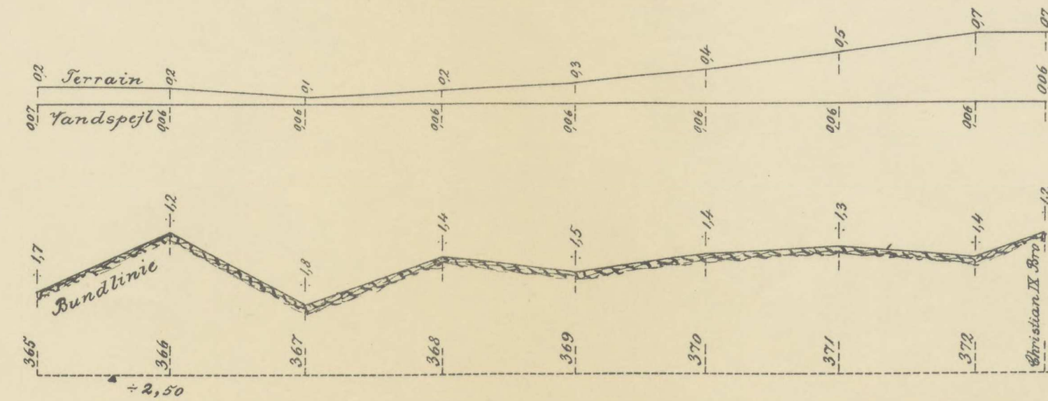
Længdeprofil 365 - Christian IX Bro. (nordre Løb).
