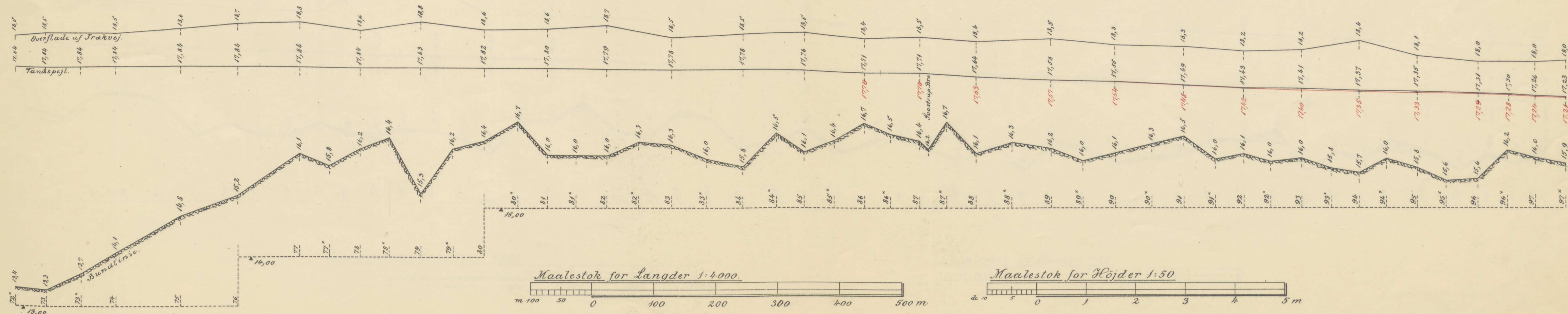
Langdeprofil 72°-97°.
