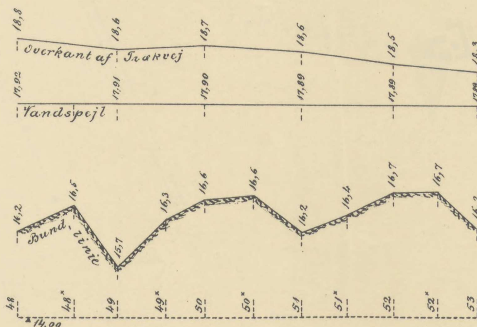
Langdeprofil 48-72.
