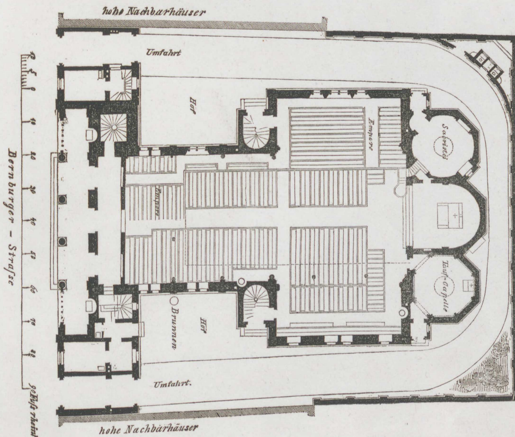
Grundriss der St. Lucaskirche.
