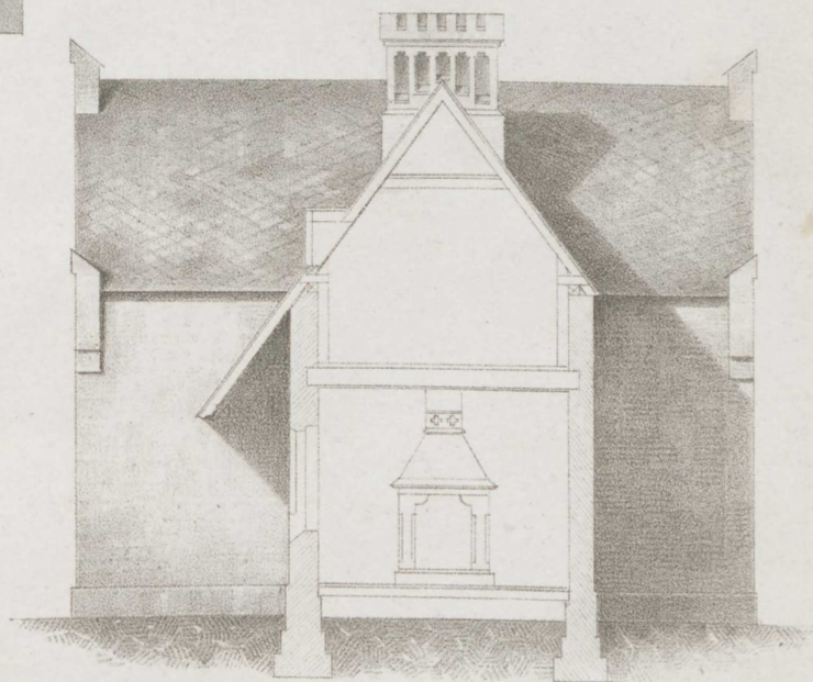
Durchschnitt nach A.B.
