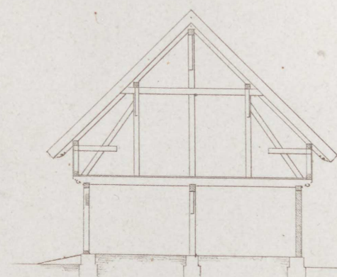
Quer-Profil der Stallung.
