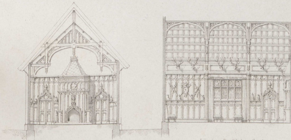
Quer Profil des Saales
