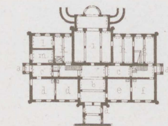
Grundriss des Unter-Geschosses.
