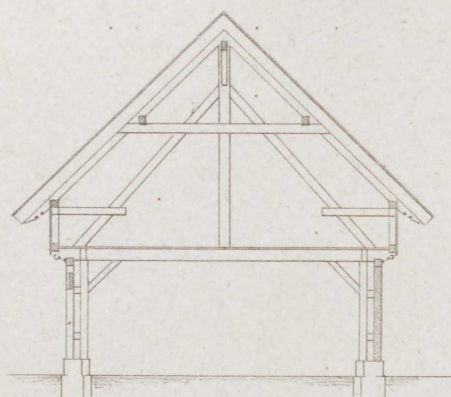
Quer Profil der Remise.
