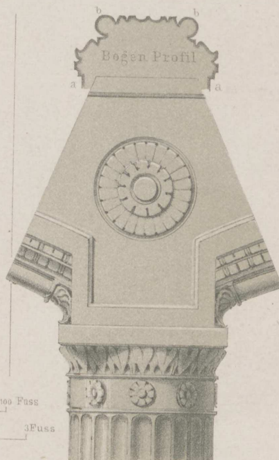
Capitell u. Bogenanfänger zur unteren Halle.
