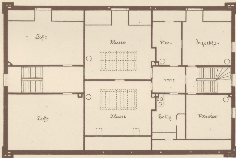
Tag-Stage
