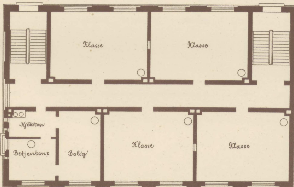
Stue Etage
