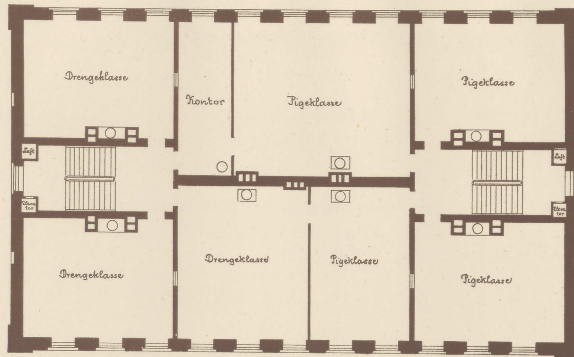
1 ste Sals Etage.
