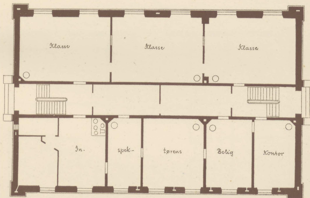
Stue - Etage
