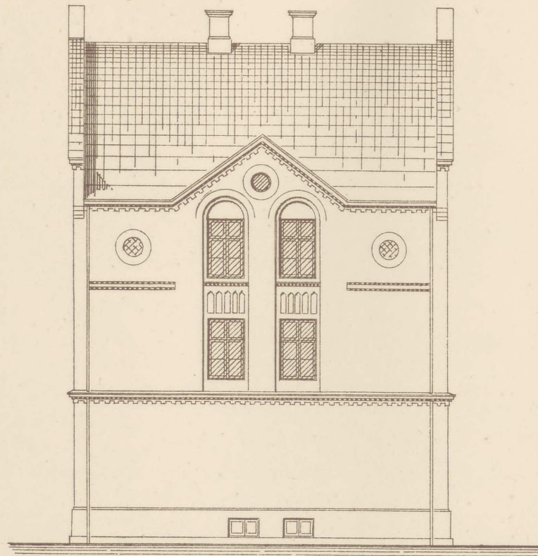
Fagade mod St. Hansgade
