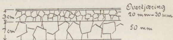
Fig. 39. Tjæremakadamisering.
