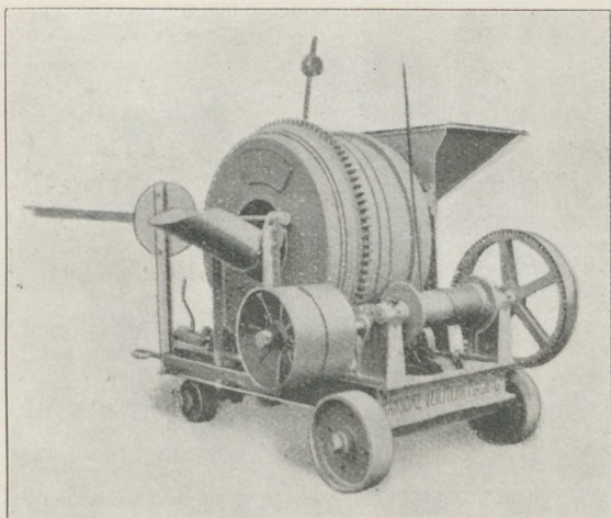
Fig. 27. Transportabel »Ransome« Maskine til mekanisk Drivkraft.
