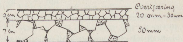
Fig. 41. Gladwellisering med Dæklag.
