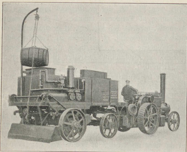
Fig. 20. Maskine, der trækkes af Lokomotiv.
