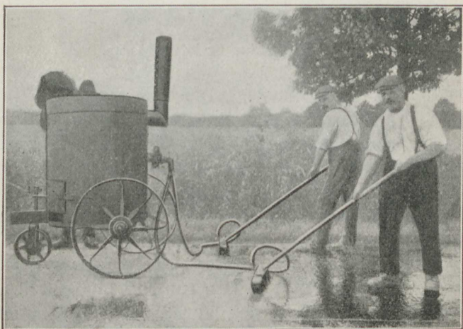
Fig. 12. Waithmanns Maskine med Koste.
