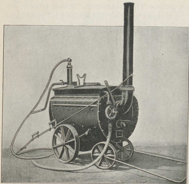
Fig. 15. Maskine med Trykspreder.
