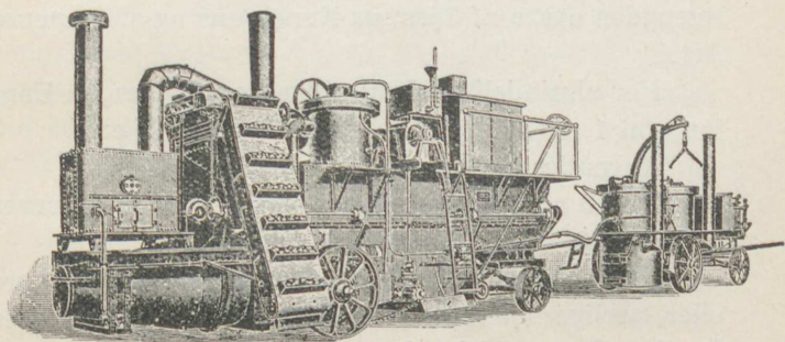
Fig. 33. Kombineret Maskine.
