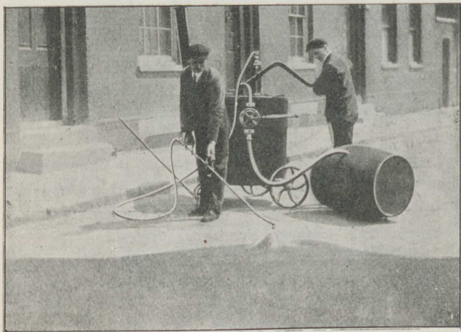
Fig. 13. Maskine med Trykspreder.
