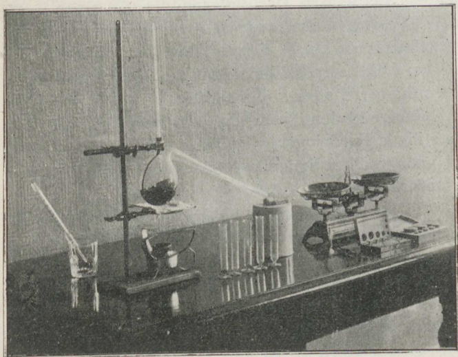
Fig. 3. Destillationsapparat.
