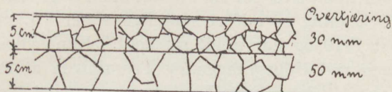
Fig. 37. Tjæremakadamisering.
