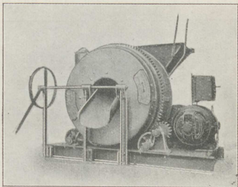
Fig. 26. Stationær »Ransome« Maskine med elektrisk Drivkraft.
