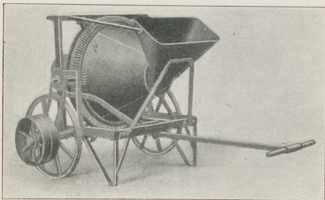
Fig. 25. »Smith« Haandblandemaskine.
