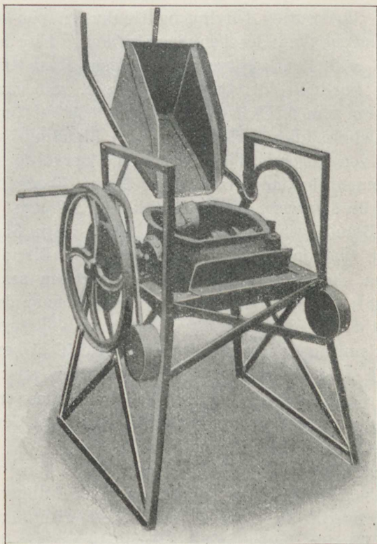
Fig. 24. »Ransome« Haandblandemaskine.
