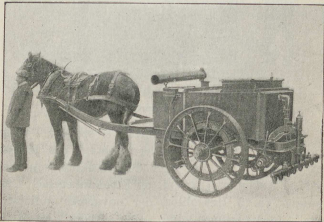
Fig. 19. Maskine med faste Trykspredere.
