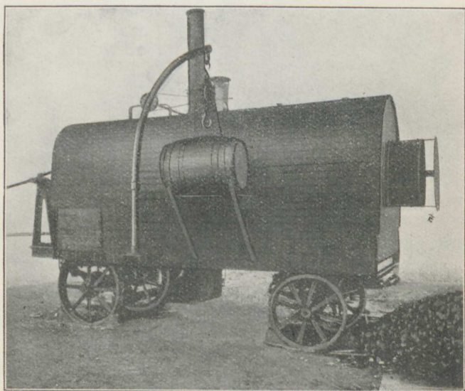
Fig. 32. »Modernmac« Maskine.
