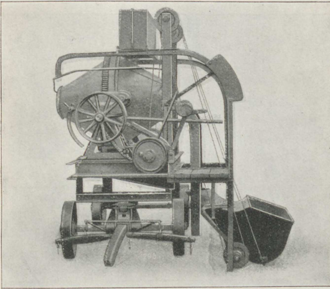
Fig. 31. »Smith« Maskine med Elevator.
