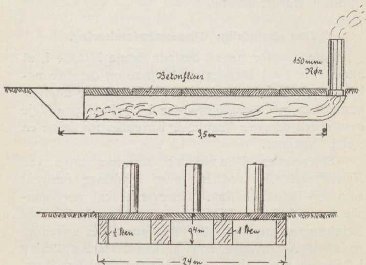
Fig. 22. Tørreovn.
