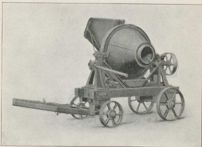
Fig. 30. Transportabel »Smith« Maskine.
