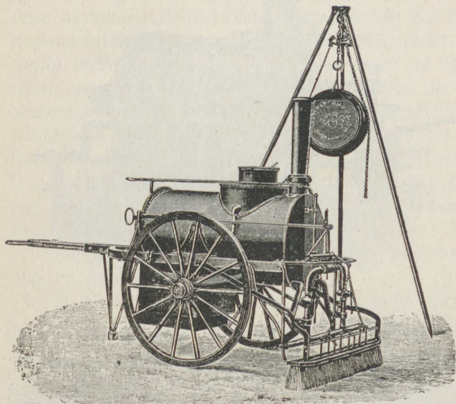
Fig. 10. Maskine med faste Koste.
