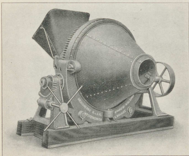
Fig. 28. Stationær »Smith« Maskine til Remtræk.
