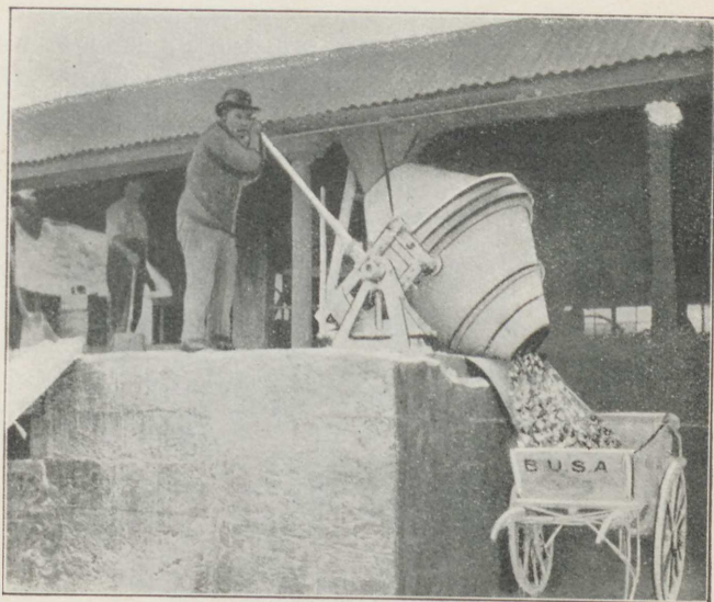
Fig. 29. »Smith« Maskinen i Virksomhed.
