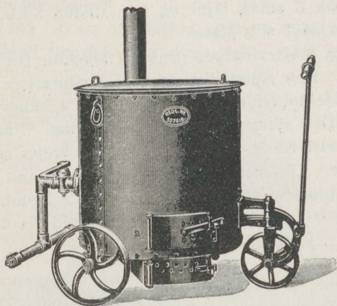
Fig. 7. Maskine med Straalerør.
