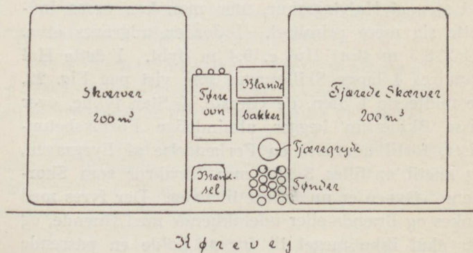
Fig. 23. Anlæg til Tjæring af Skærver.
