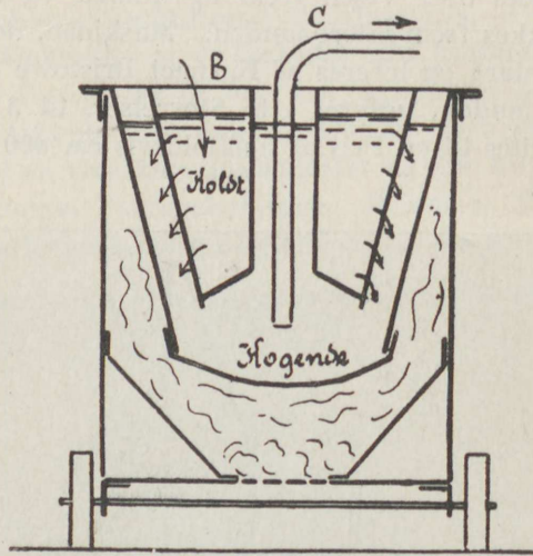
Fig. 18. Maskine med Cirkulationsbeholder.
