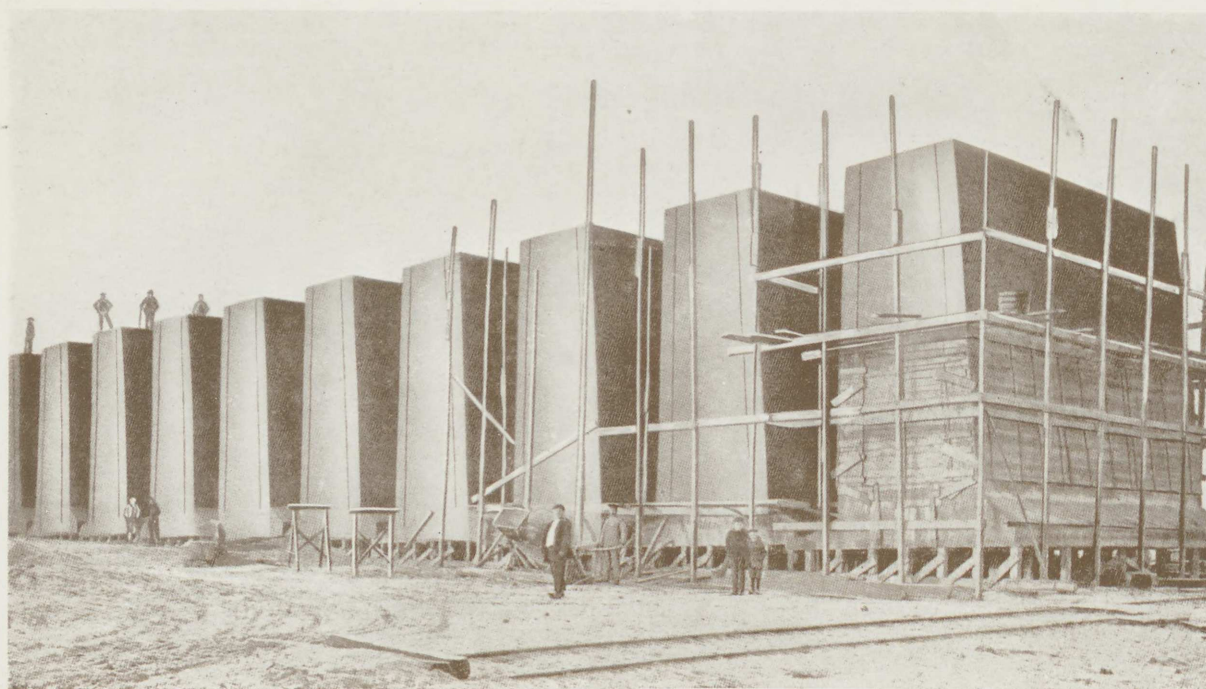
SÆNKEKASSER PAA STABELEN.
