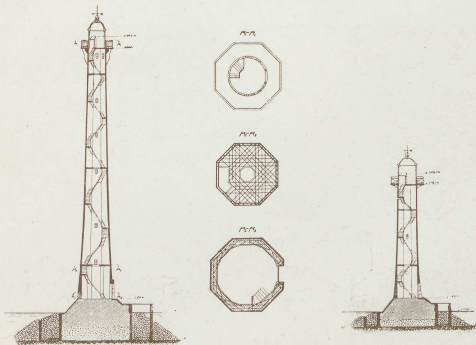
FYRTAARNE I KANALEN MELLEM PETROGRAD OG KRONSTADT.
