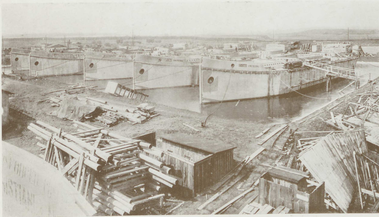
5 1000 TONS KULBAADE FLOT I VOR TØRDOK I TILBURY. Bygherre: DET BRITISKE ADMIRALITET.
