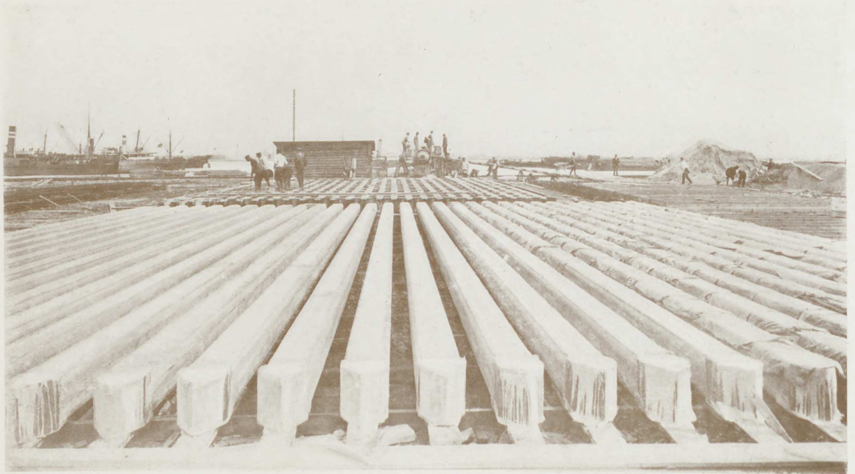
PÆLESTØBNING.
