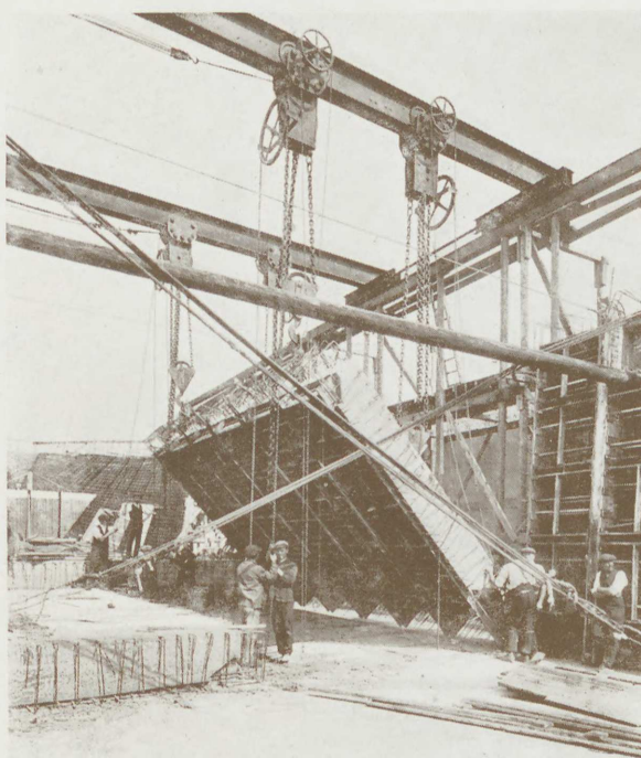
1000 TONS KULBAADE UNDER BYGNING. Siderne løftes.
