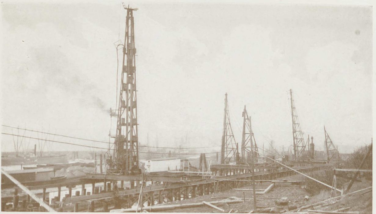
PÆLERAMNING.
