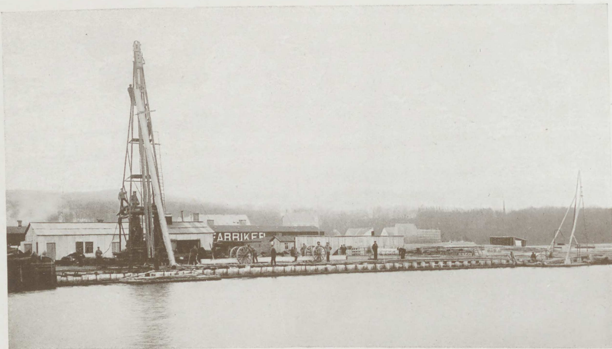
BOLVÆRK VED RANDERS, DANMARK.
