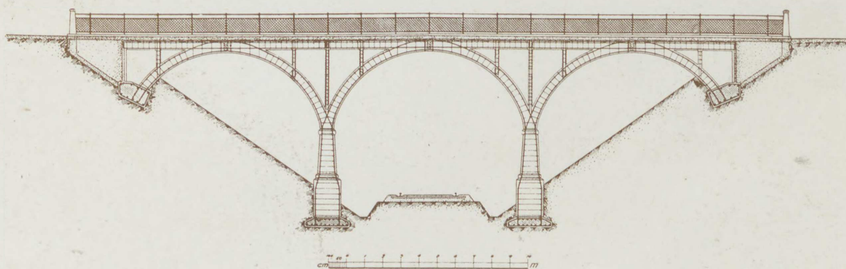
VIADUKT MELLEM VEJLE OG HORSSENS, DANMARK.
