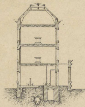
Snit A. B. 1:500
