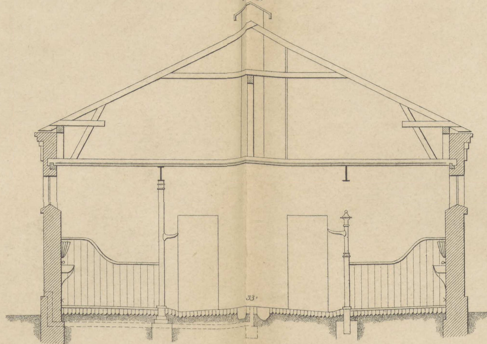
Fig 11. 1:100.
