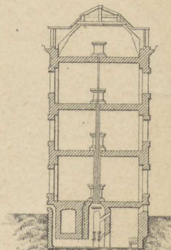
Snit C. D. 1:500
