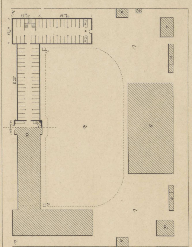
Fig 2 1:1000
