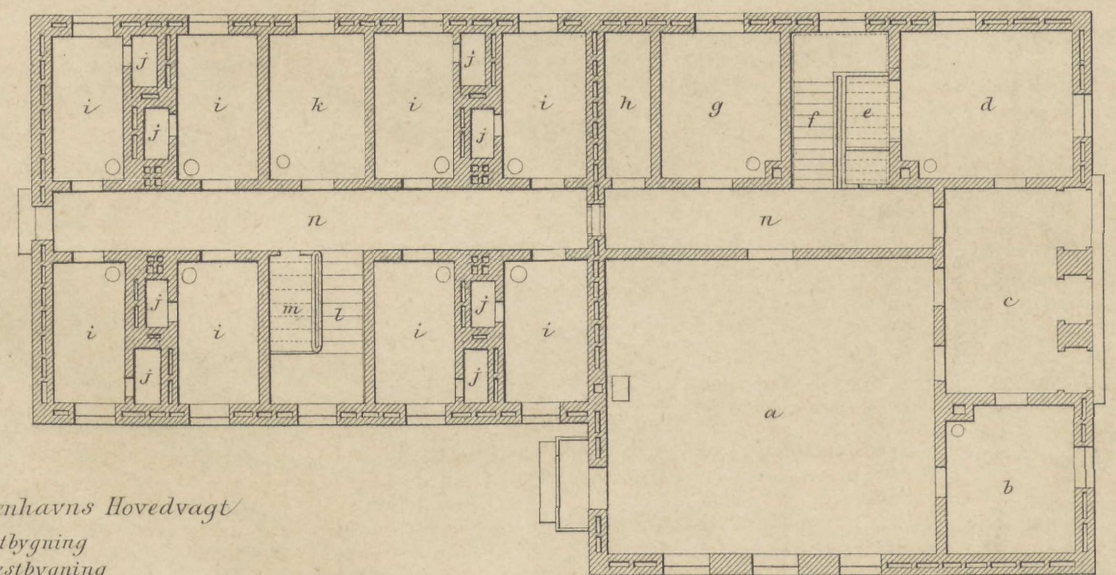
Fig 3 1:200
