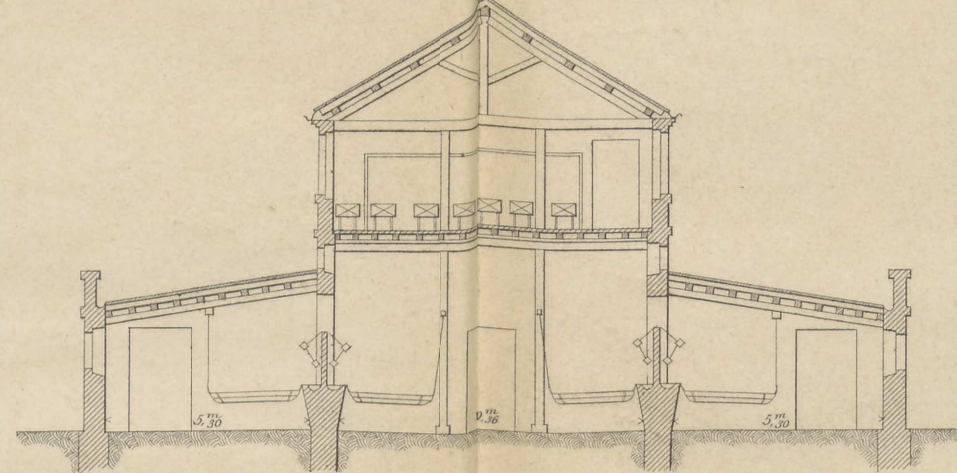
Fig 10 1:200.
