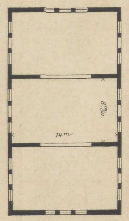
Fig 6 1:500
