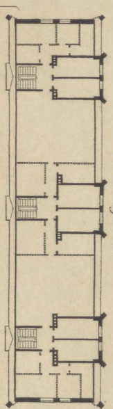
Fig 1 Loftsetage (1.500)
