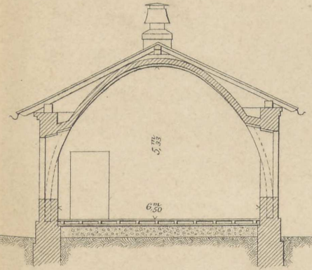
Fig 10 1:200.
