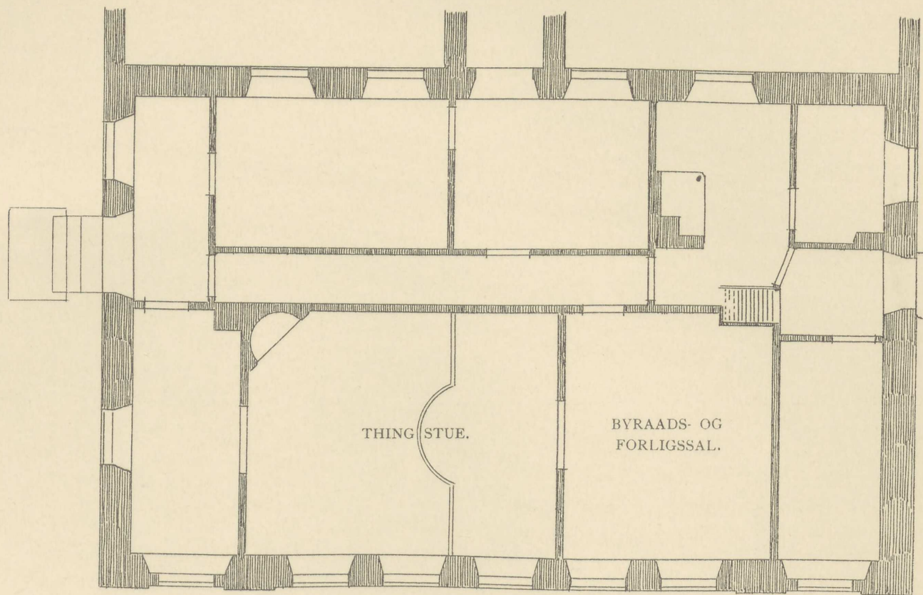
STUEPLAN.
