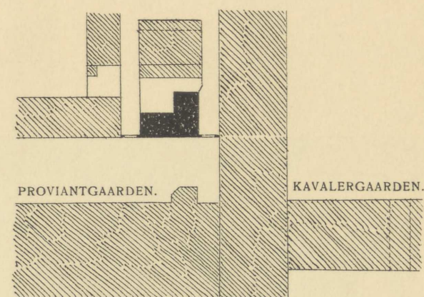
BELIGGENHEDSPAN 1:1000.
