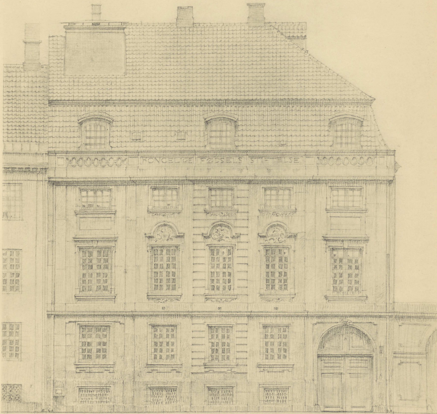
SIDE MOD AMALIEGADE.
