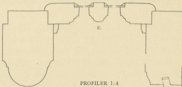
PROFILER 1:4
