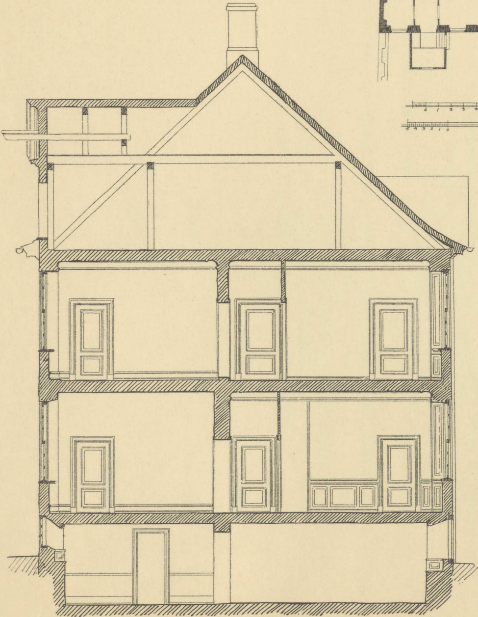
TVÆRSNIT
