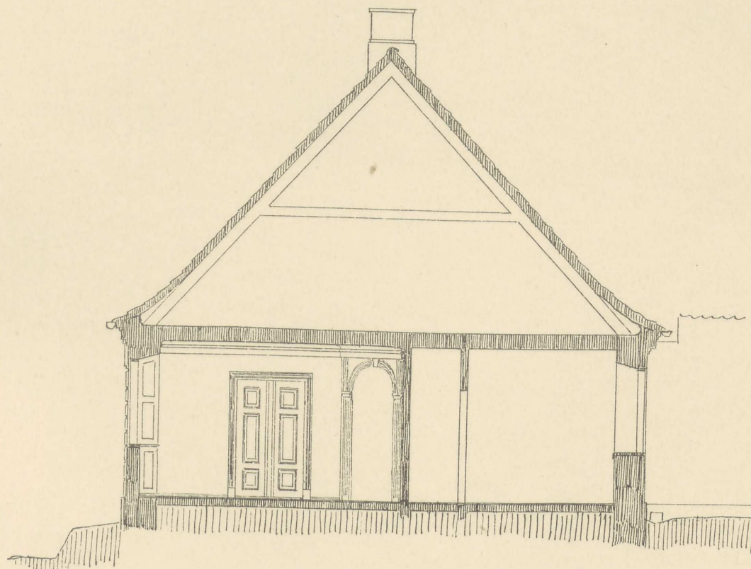
TVÆRSNIT.
