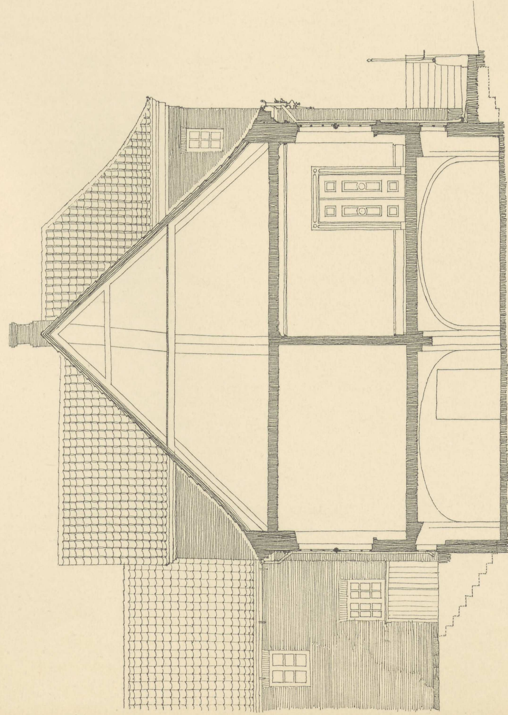
TVÆRSNIT
