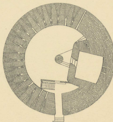
GRUNDPLAN
