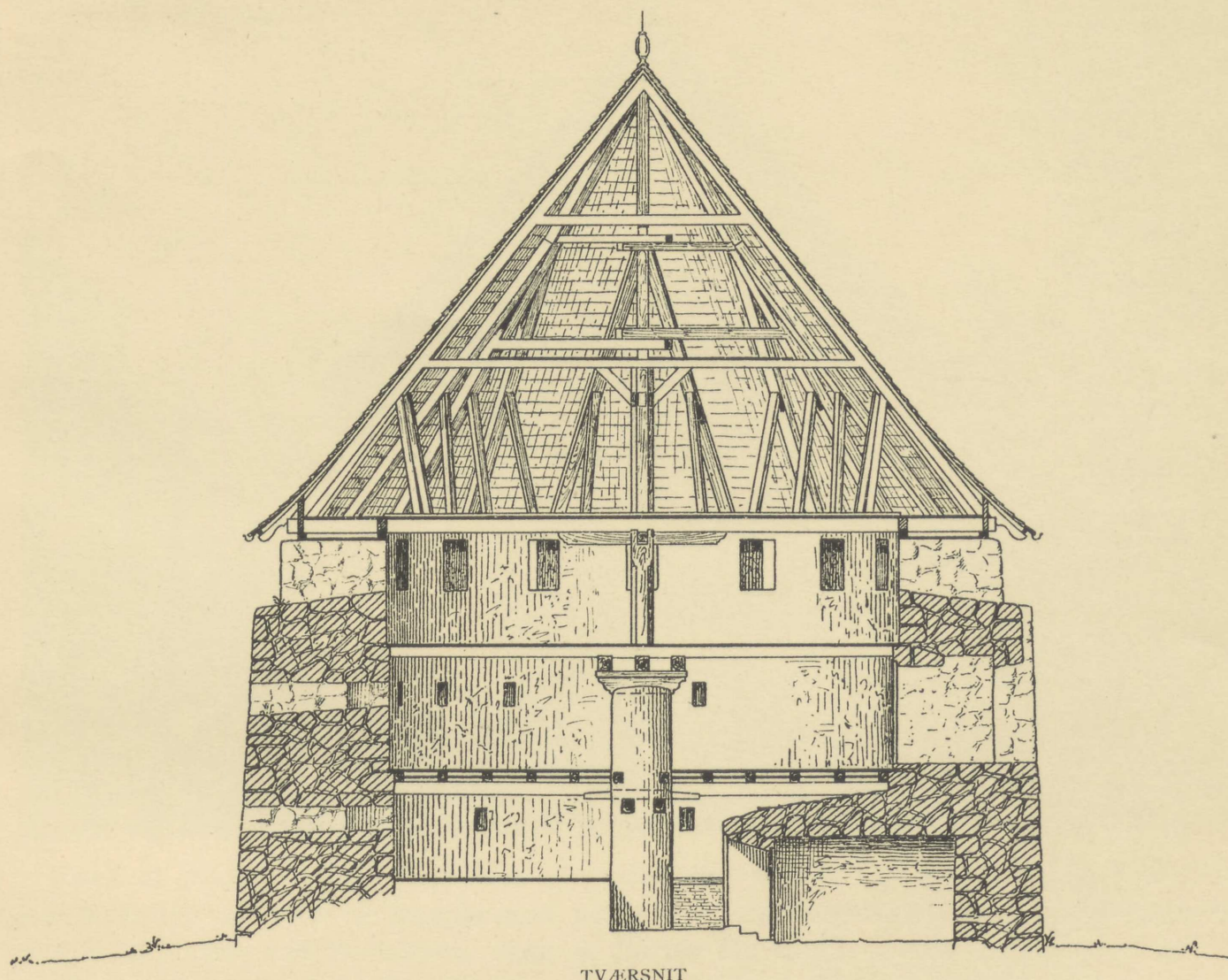
TVÆRSNIT
