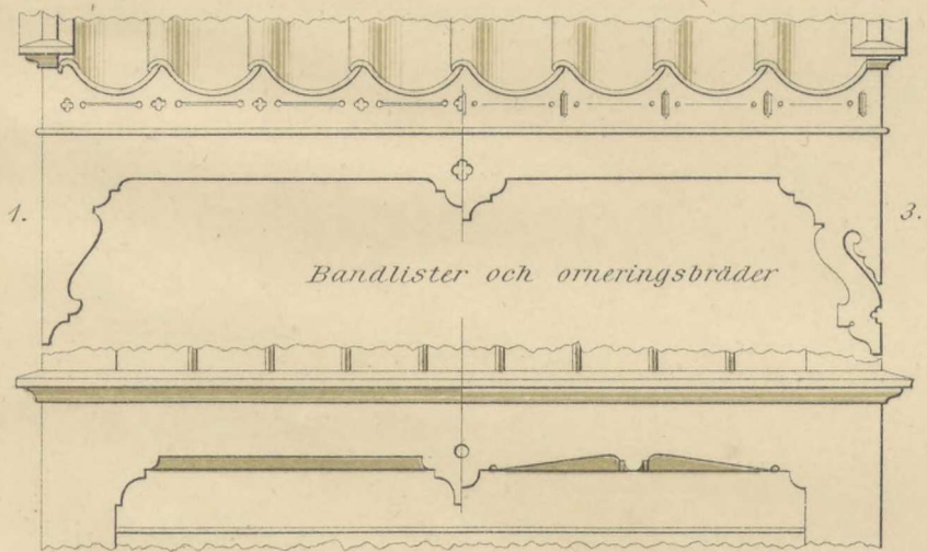
Ornering för brädbeklädnad å yttre väggar.
