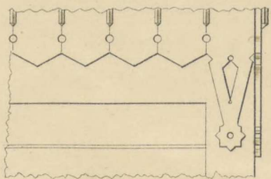
Bandlister och orneringsbräder för brädbeklädnad å yttre väggar.
