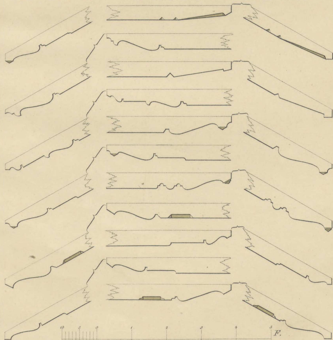
Sparrhufvud å sidor.
