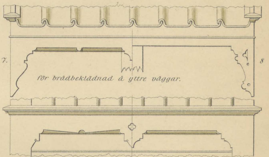
Ornering för brädbeklädnad å yttre väggar.
