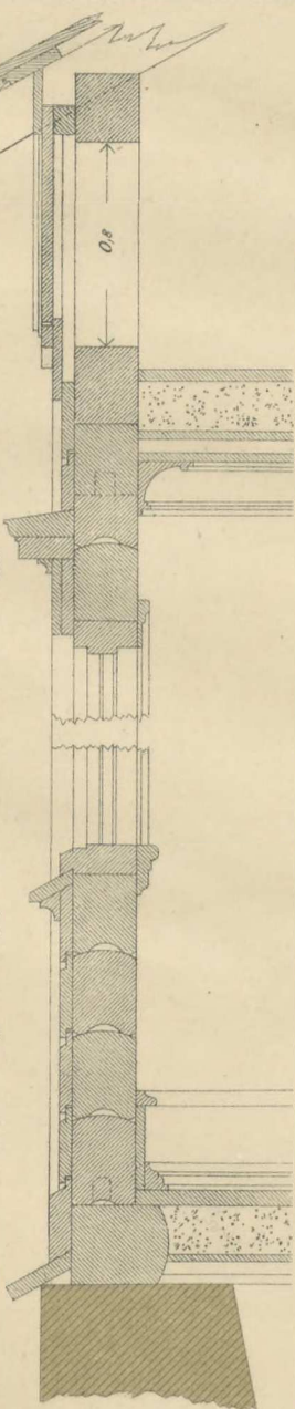
Genomskärning af vägg med stående timmer. Liggande under fönster.
