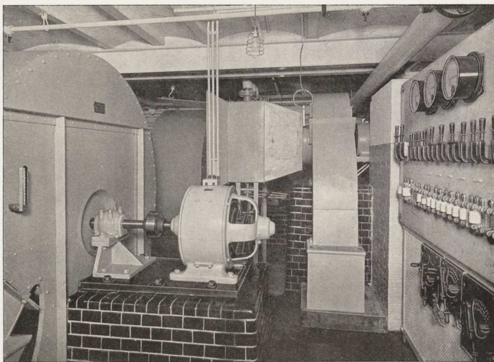
LUFT DYNAMO
