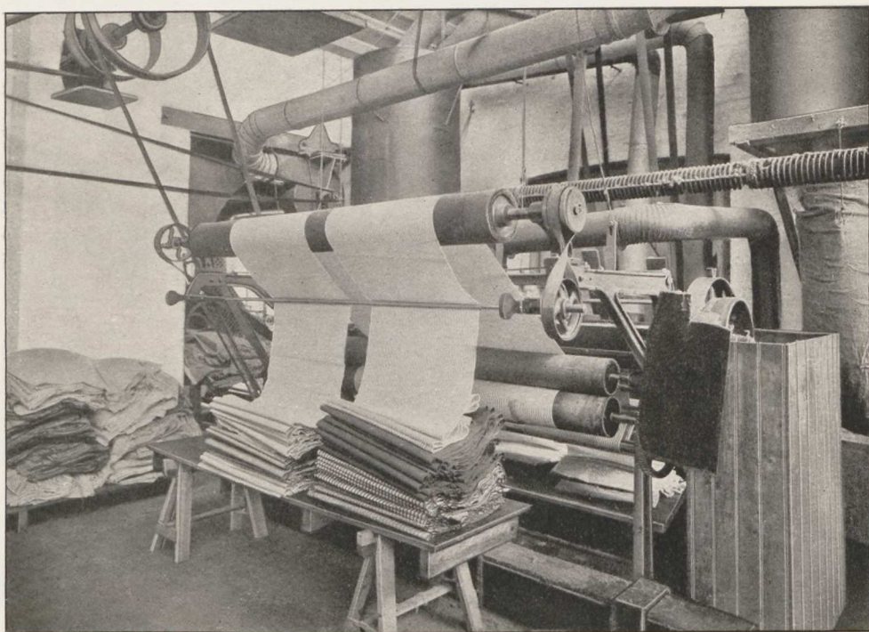
SKÆREMASKINE
