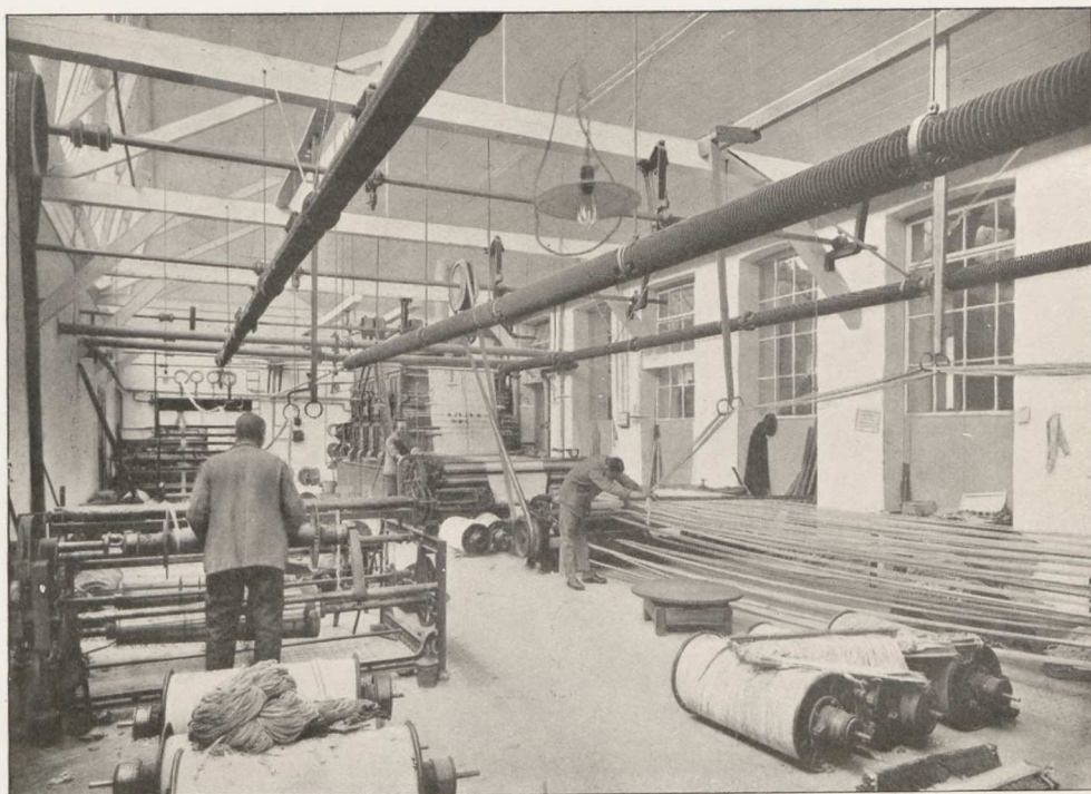
KÆDESKÆRERI
