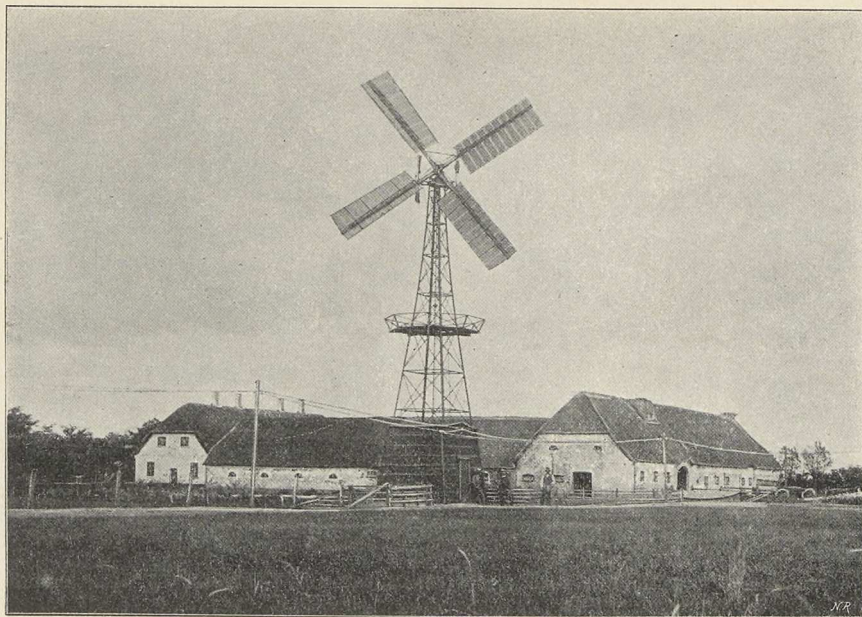
Fig. 1. J. Boesens Gaard og Mølle, i Askov.
