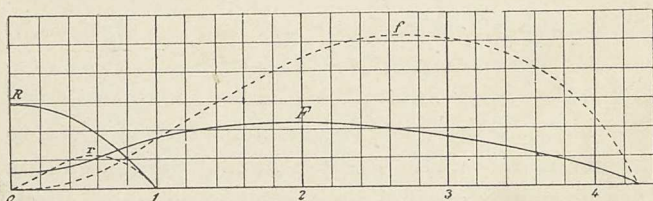
Fig. 5. Tryk paa en Plade med 10^{\circ} Heldning ( F ) og 45^{\circ} Heldning ( R ) ved forskellige Hastigheder, og de dertil svarende Arbejdsevner ( f og r ).
