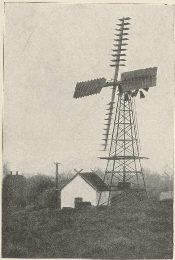
Fig. 6. Mølle ved et Landsbyværk i Vallekilde.
