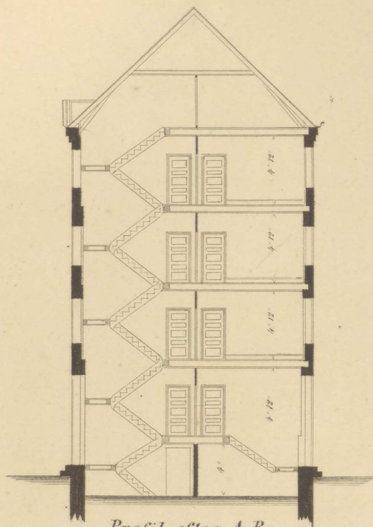
Profil efter A.B.
