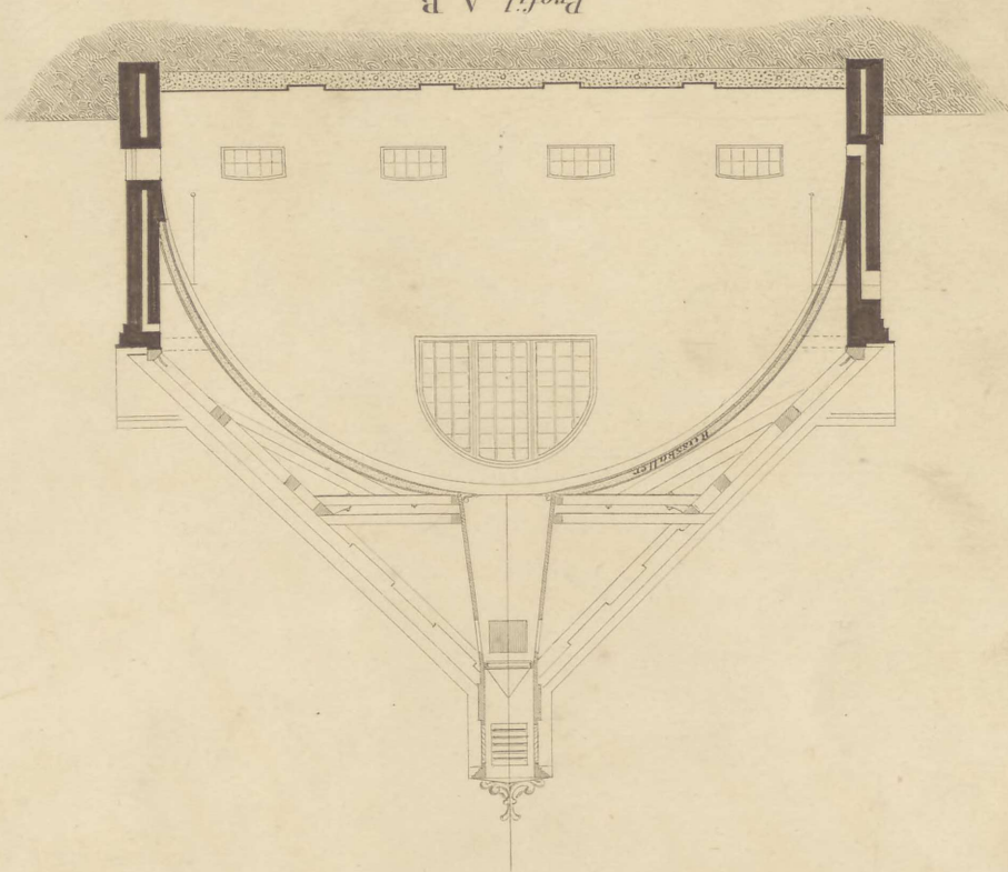
Profil A B
