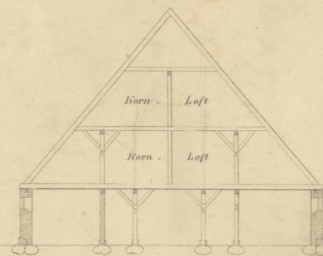
Profil af Stalden efter Linien a b.
