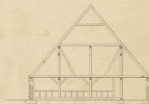
Profil af samme efter Linien c d.
