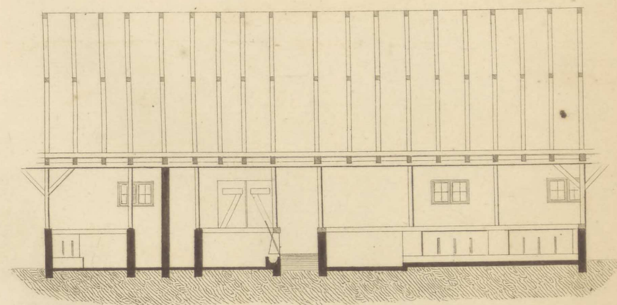
Profil C D
