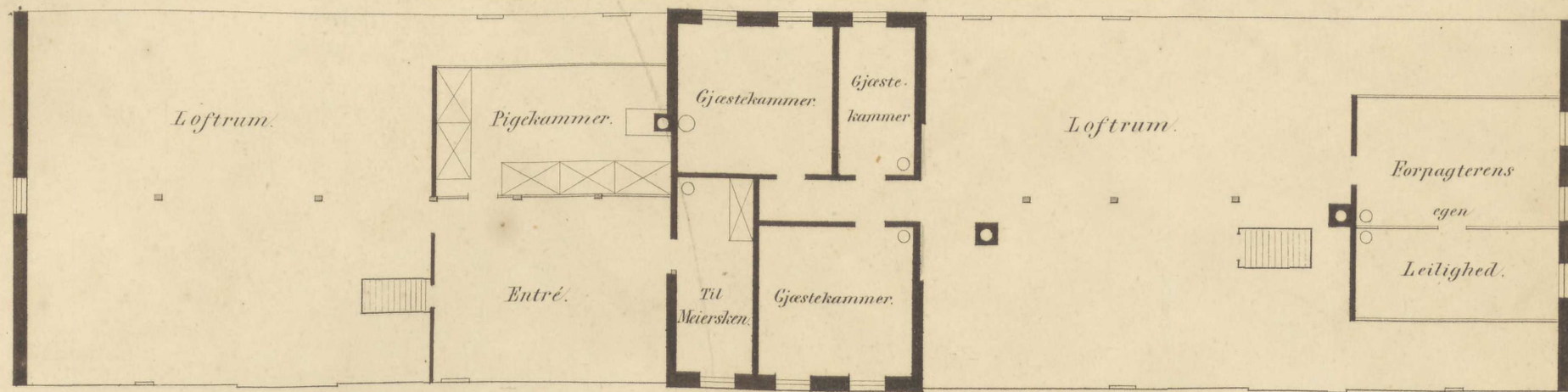
Plan af øverste Etage.
