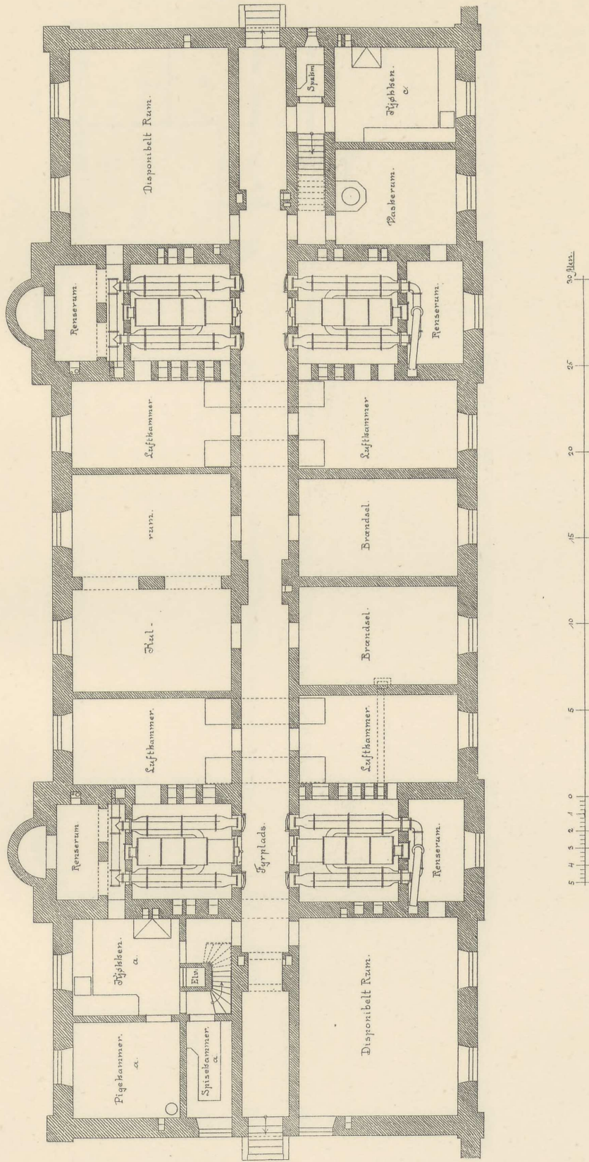
Plan of Skjælderens.
