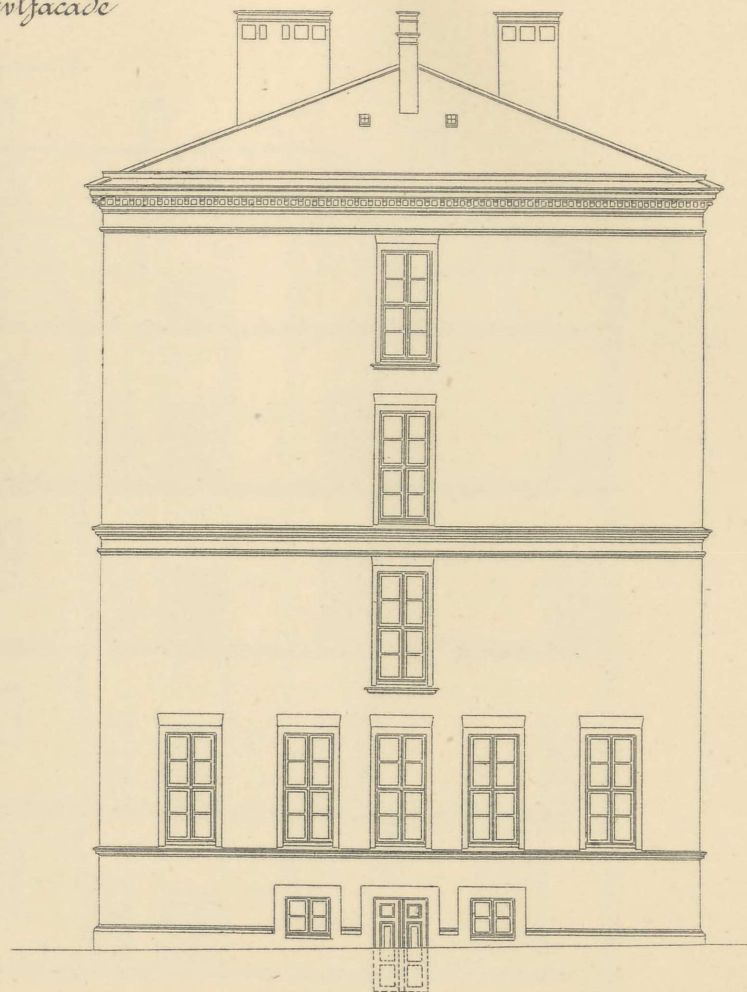
Sværmitt & Gavlfacade
