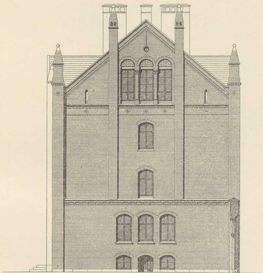
Gavl mod Øst ·
