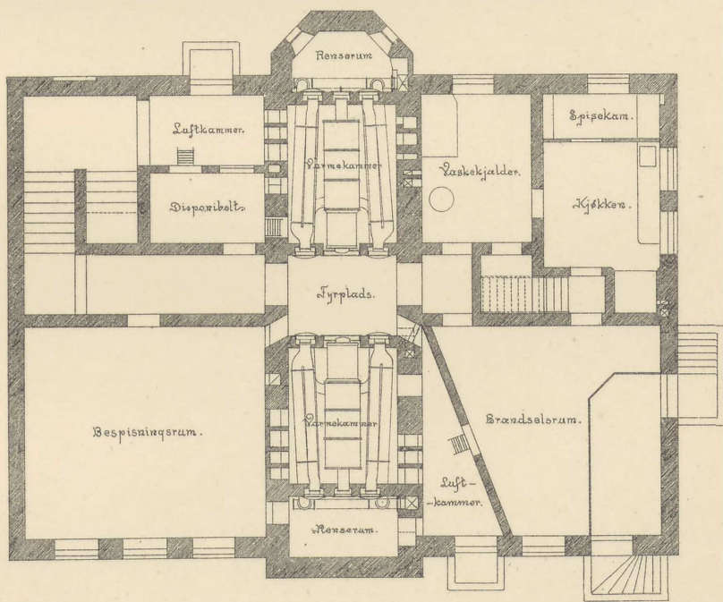
Plan af Kjælderen.
