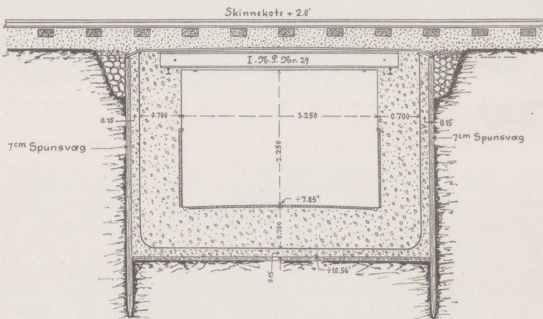
Fig. 32. Tværnsnit af Perrontunnel.
