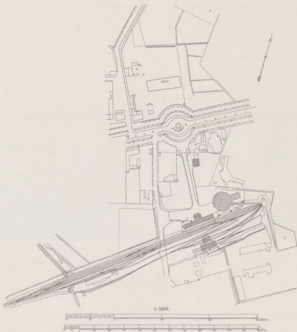
Fig. 2. Banegaardsterrainet 1847—1864.
