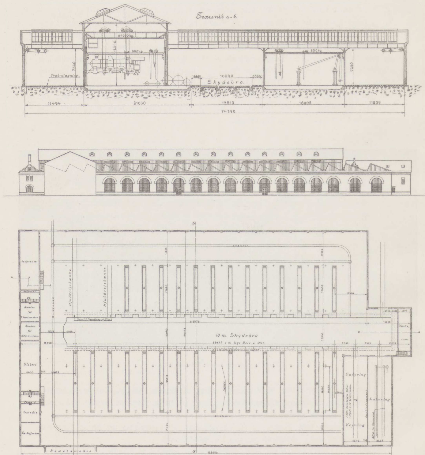
Fig. 53. Lokomotivreparationsværkstedet.
