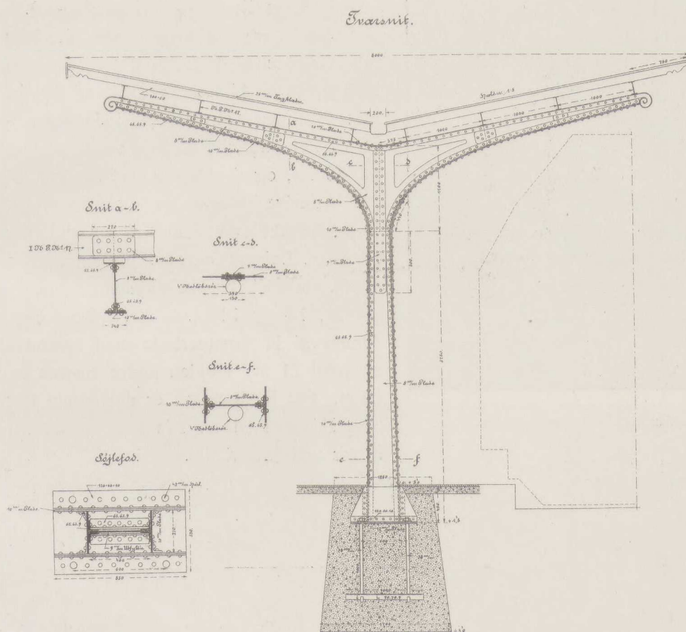
Fig. 39. Tage over Postperroner.
