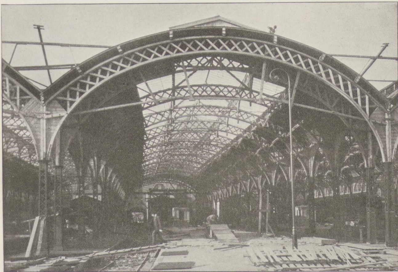
Fig. 33. Perronhal.
