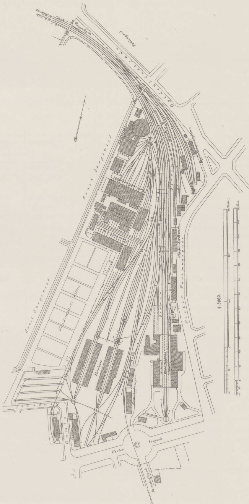
Fig. 4. Banegaardsterrænet 1864—1911.
