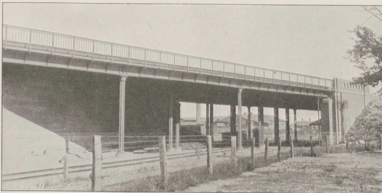
Fig. 75. Viadukt over Godsbanen.
