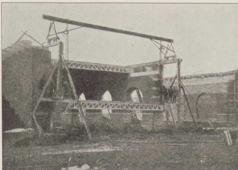
Fig. 84. Viadukten for Tagensvej. Monteringskran.
