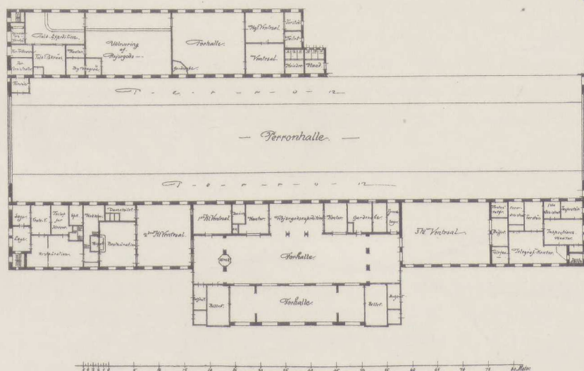
Fig. 6. Plan af Banegaardens Hovedbygning.
