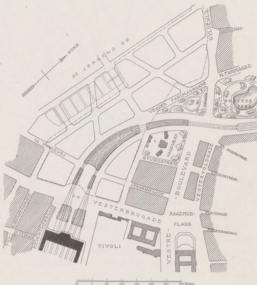
Fig. 21. Det fuldstændige Projekt af November 1901. Gadeordning omkring Frihedsstøtten.
