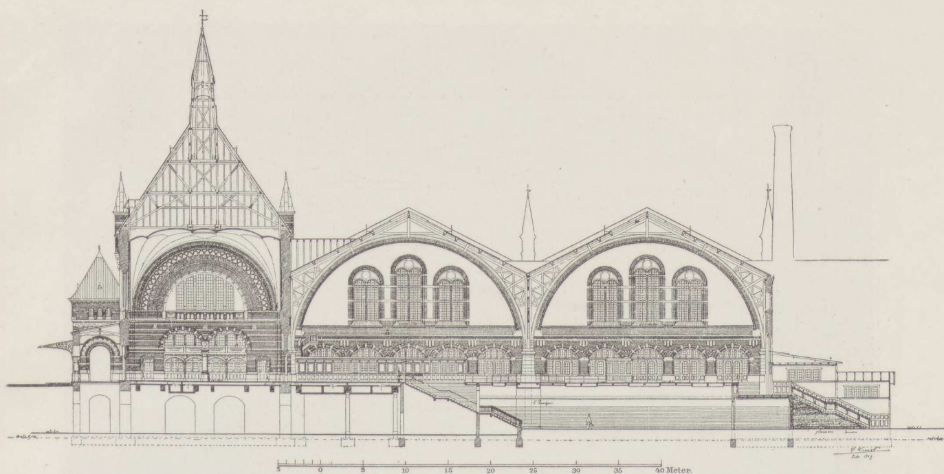
Fig. 28. Den nye Hovedbygning. Tværsnit.
