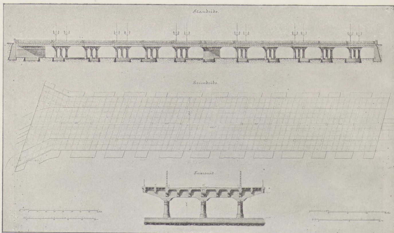
Fig. 34. Tietgensgadeviadukten.
