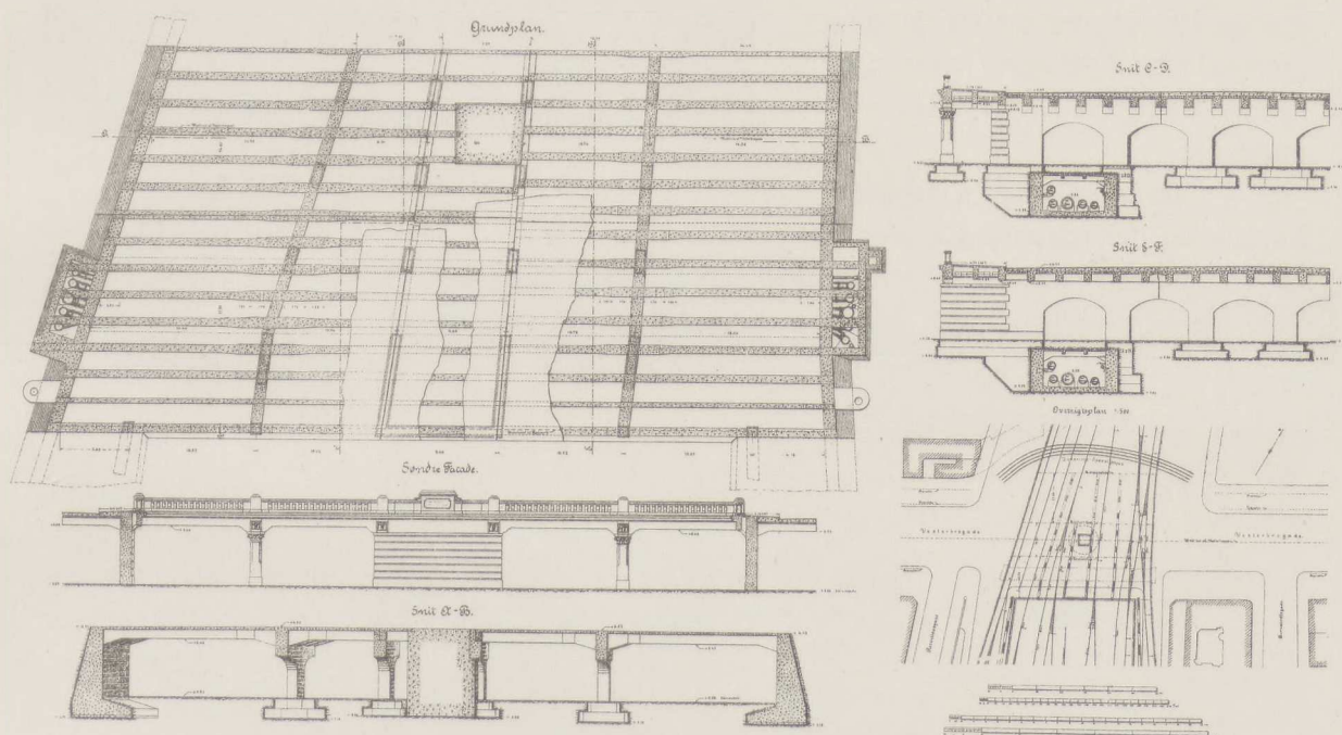
Fig. 66. Viaduktanlæg for Vesterbrogade.
