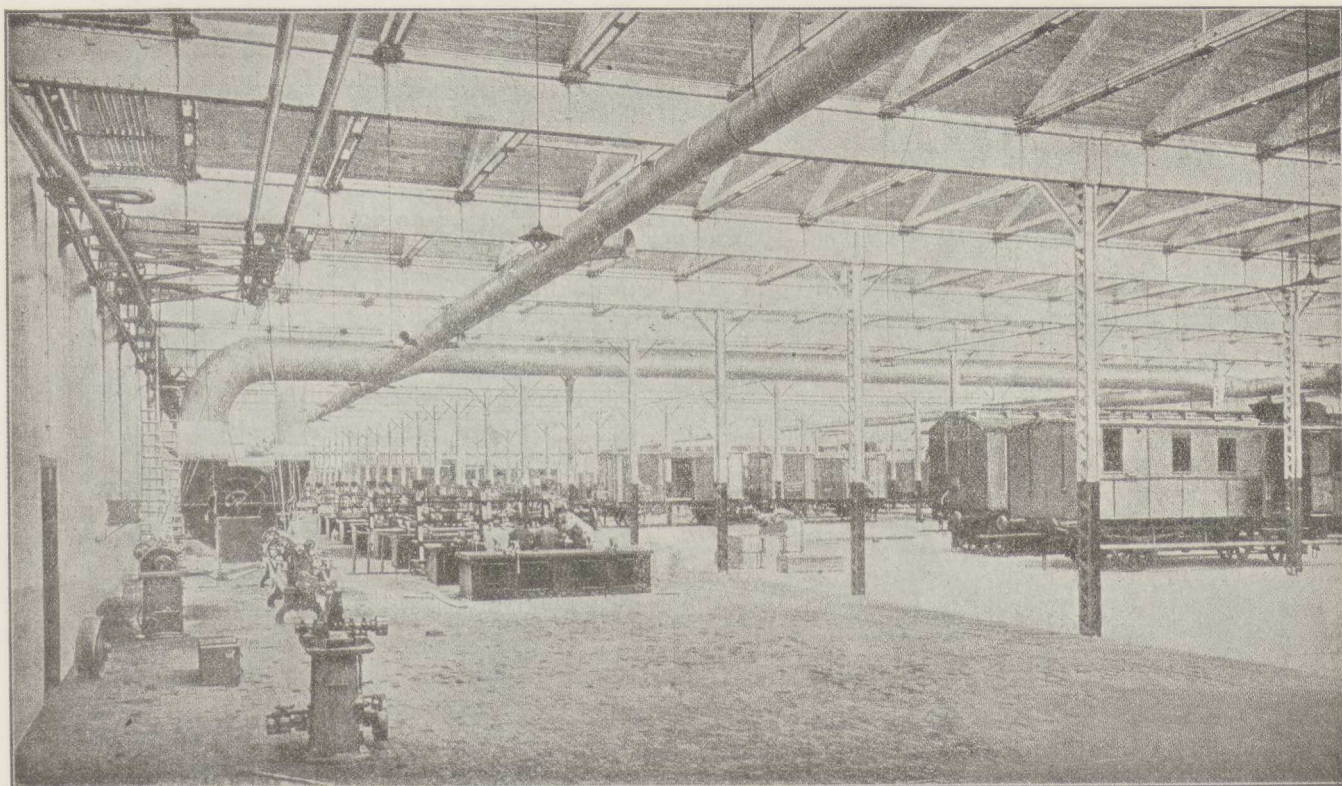
Fig. 54. Vognreparationsværkstedet.
