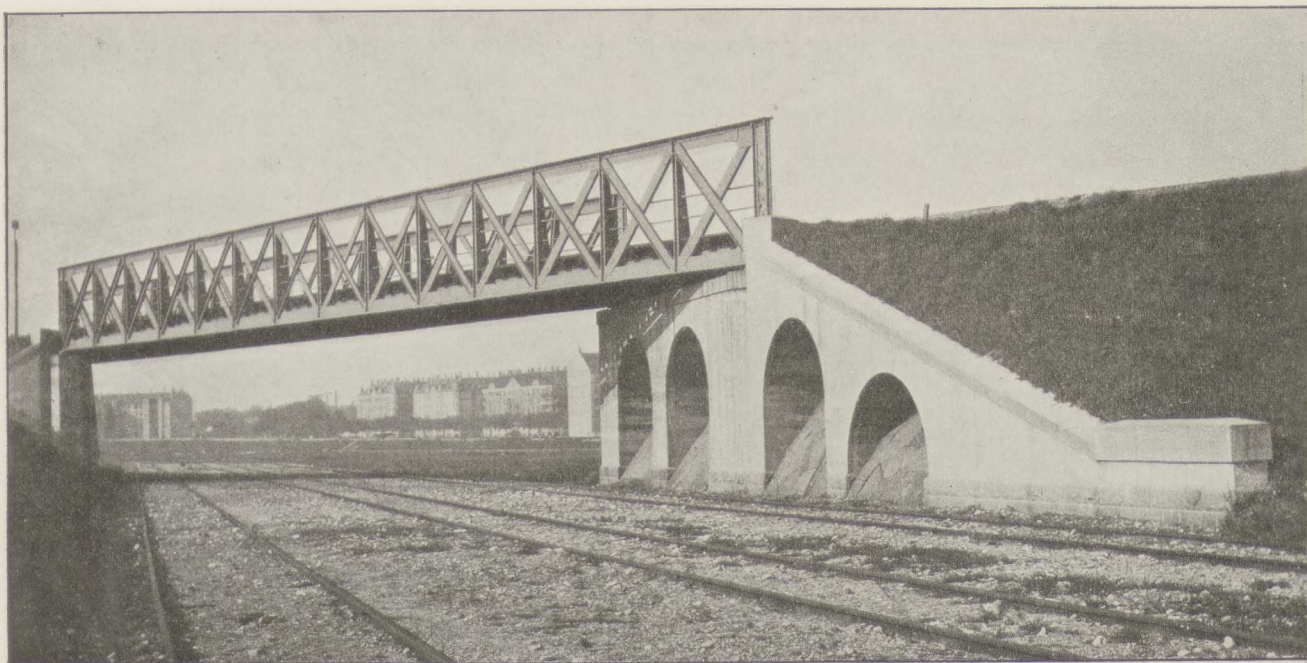
Fig. 46. Enkeltsporet Lokomotivviadukt.
