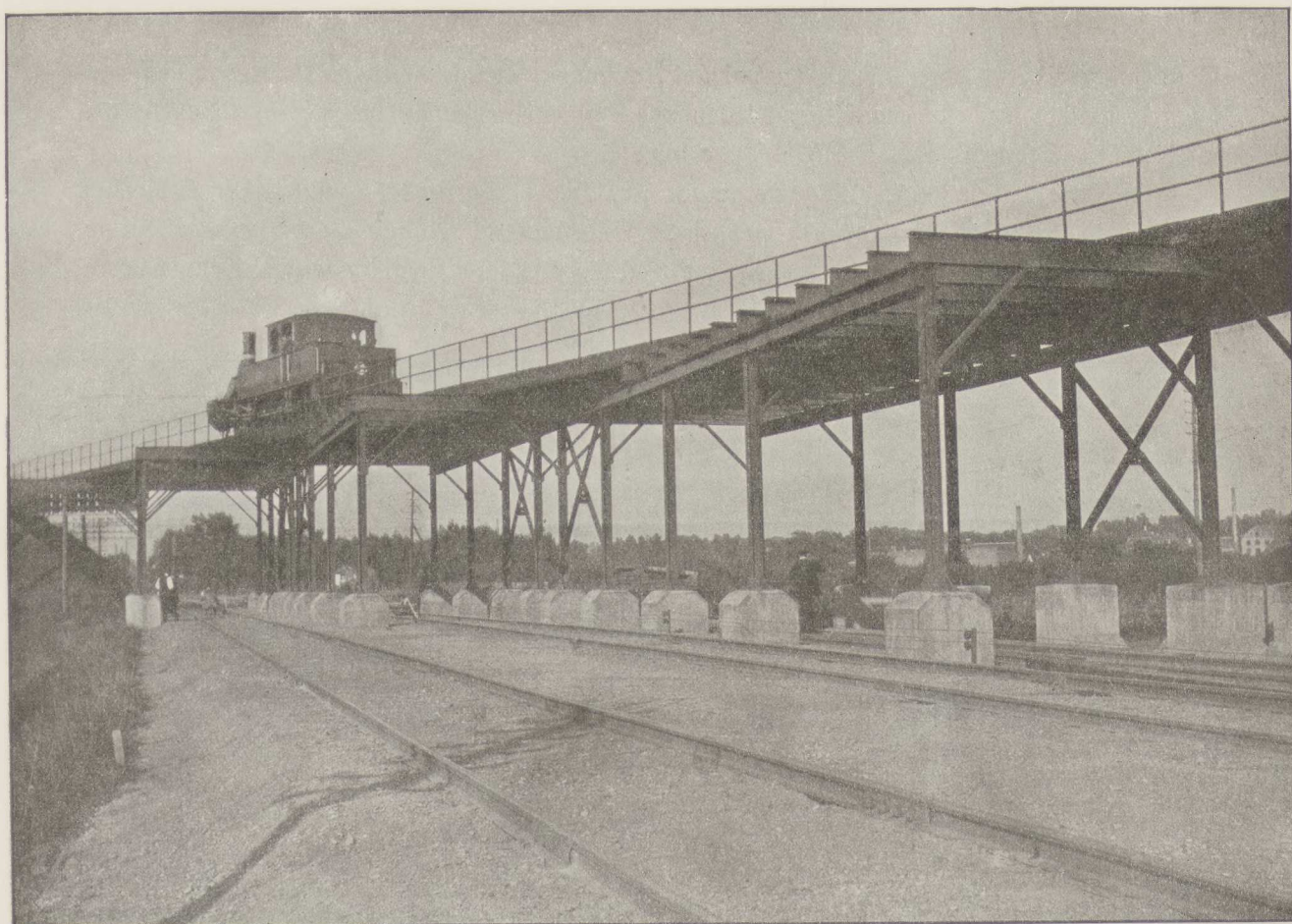
Fig. 89. Viadukten over Vestbanen.
