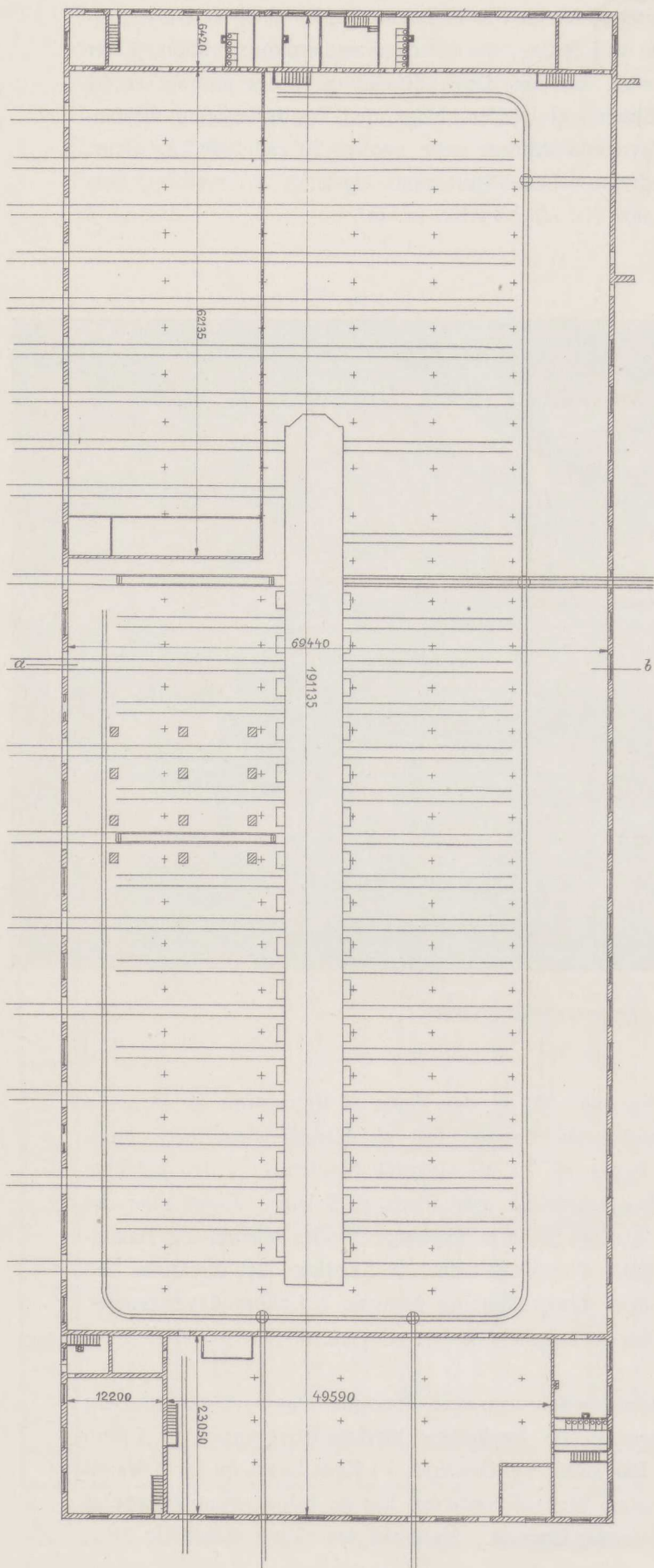
Fig. 55. Vognreparationsværkstedet.
