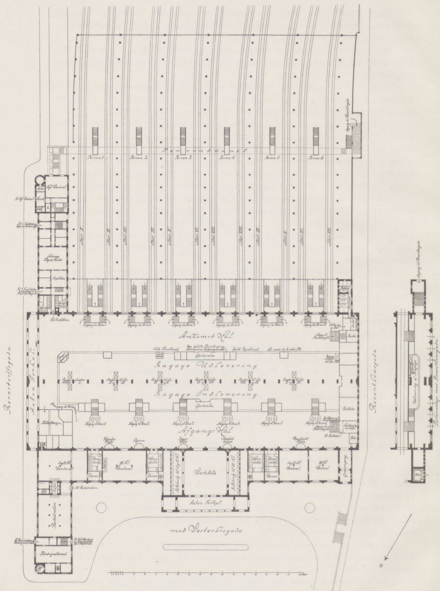
Fig. 27. Den nye Hovedbygning. Grundplan.
