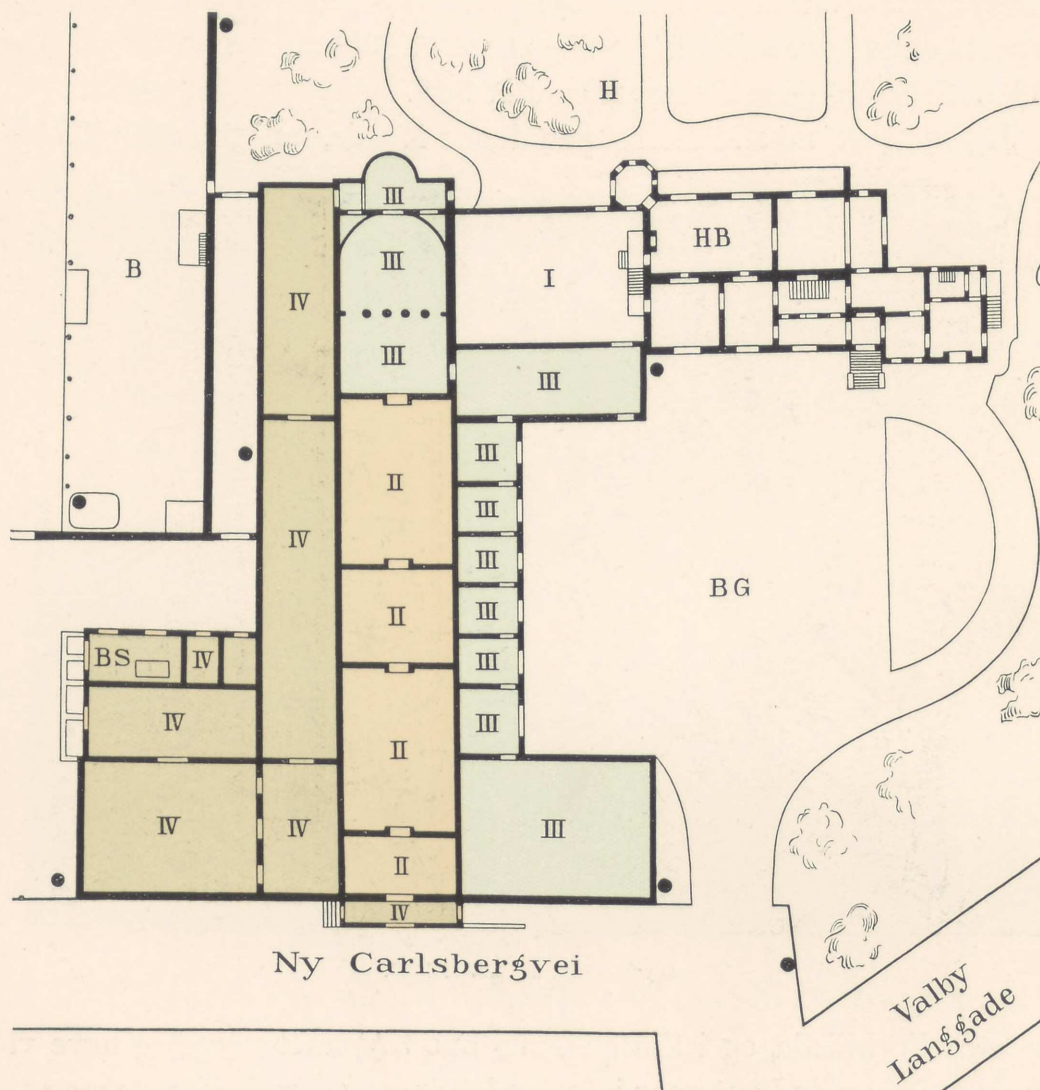
Plan af Ny Carlsberg Hovedbygning og Glyptotek 1896.
