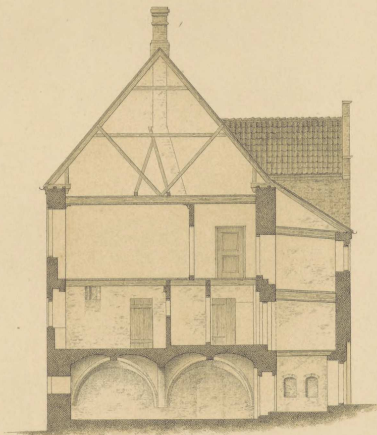
Tværsnit.
