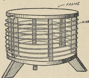
FIG. 48.—Helix.
