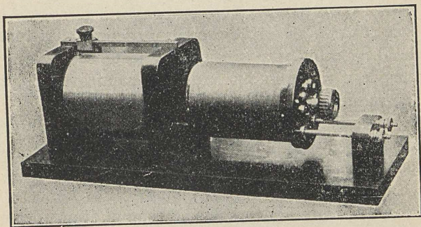
FIG. 92.—Loose coupled tuner.
