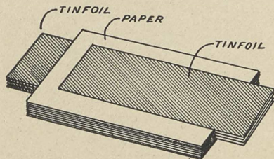
FIG. 80.—Fixed condenser.
