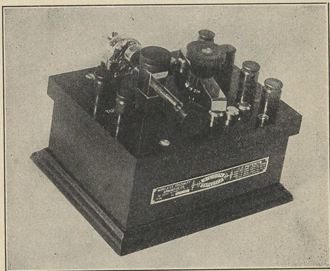
FIG. 70.—Perikon detector.
