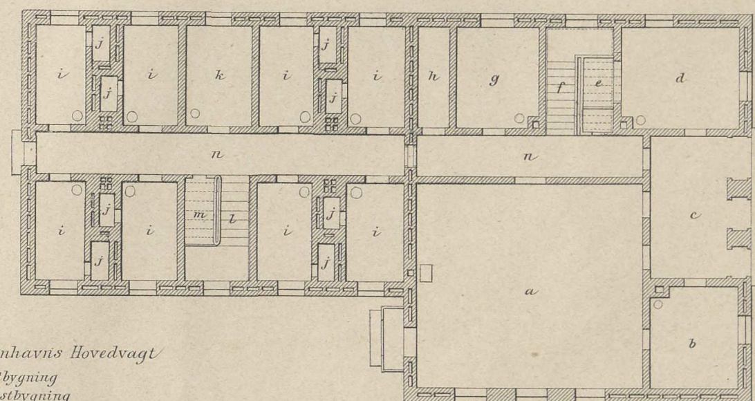
Fig 3 1:200
