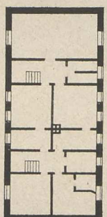
Fig 8 1:500
