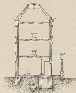
Snit A.B. 1:500
