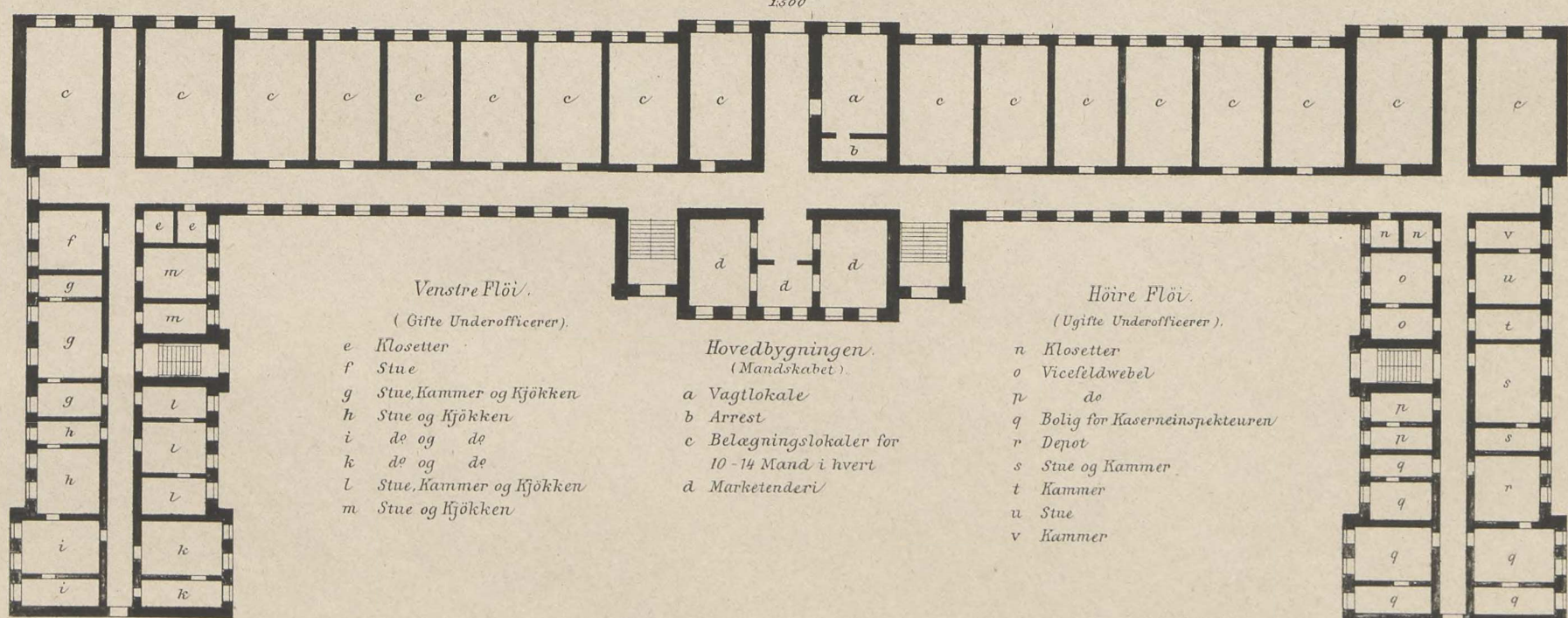
Fig 10. 1:300
