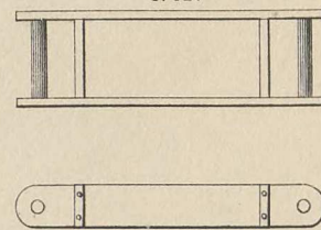
fig 4. 1: 12.
