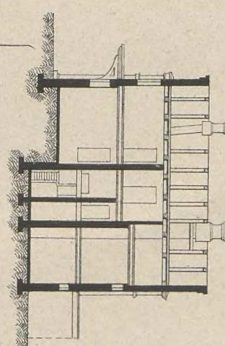
Fig 6 1:500
