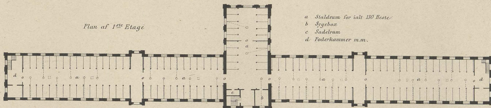
Fig 5 1:500
