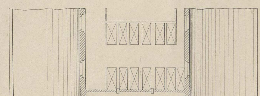
Fig 7 1:200.
