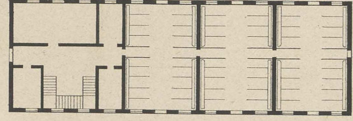
Fig 4a 1ste Etage (1:500)
